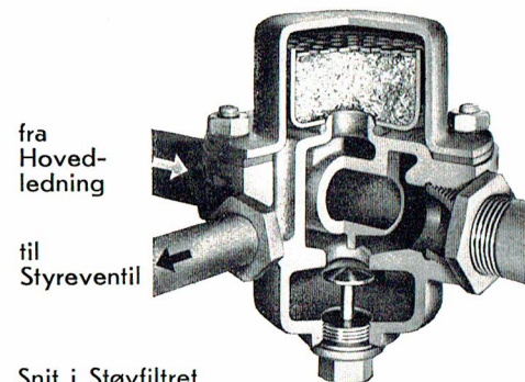
Fig. 84 Snit i Støvfiltret
