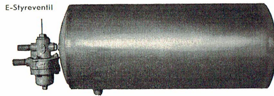
Fig. 60 Hjælpeluftbeholder med E-Styreventil for Lokomotiver
