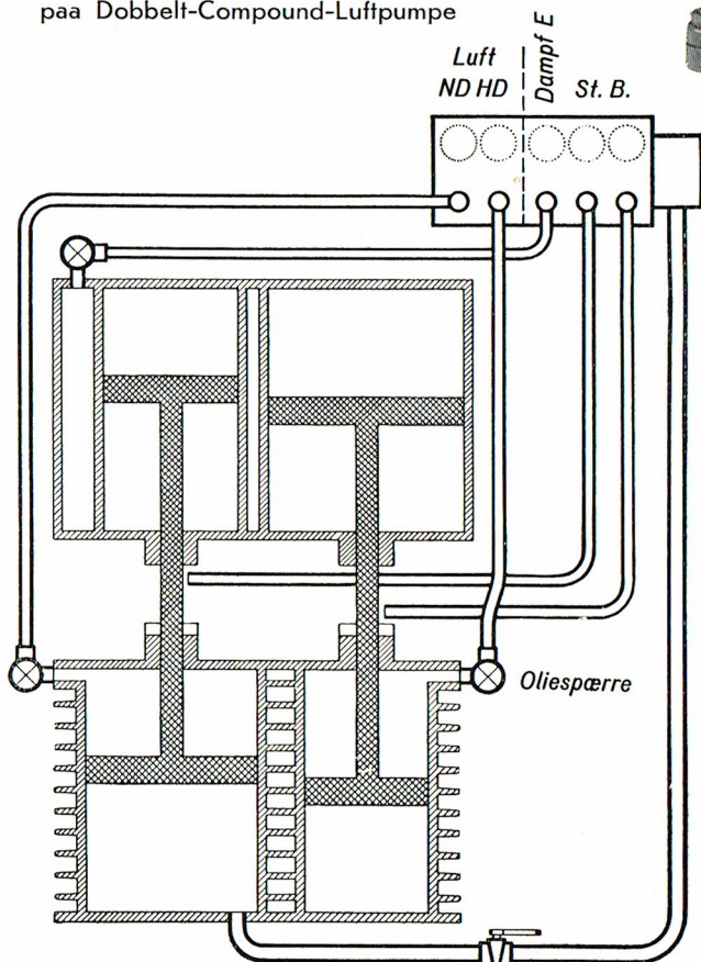
Fig. 30 Smøreplan for en Dobbelt-Compound- Luftpumpe med Smørepumpe KL 5
