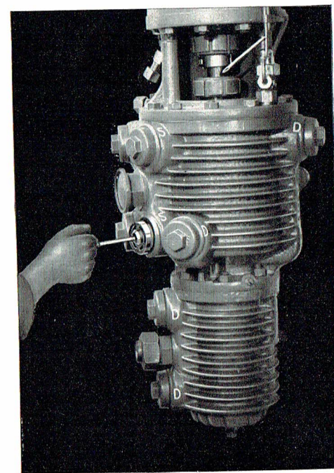
Fig. 12 Indbygning af en Pladeventil
