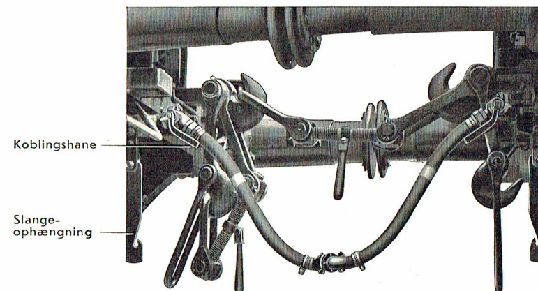
Fig. 68 Bremsekoblingerne samlet
