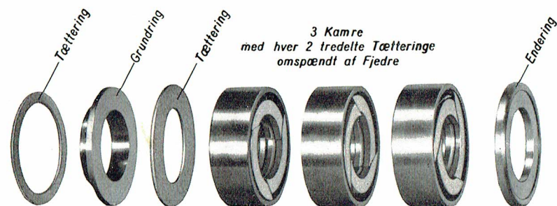
Fig. 19 En Metalpaknings enkelte Dele
