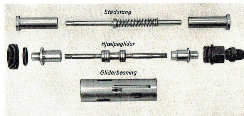
Fig. 23 Nielebock-Hjelpestyringens Enkeltdele
