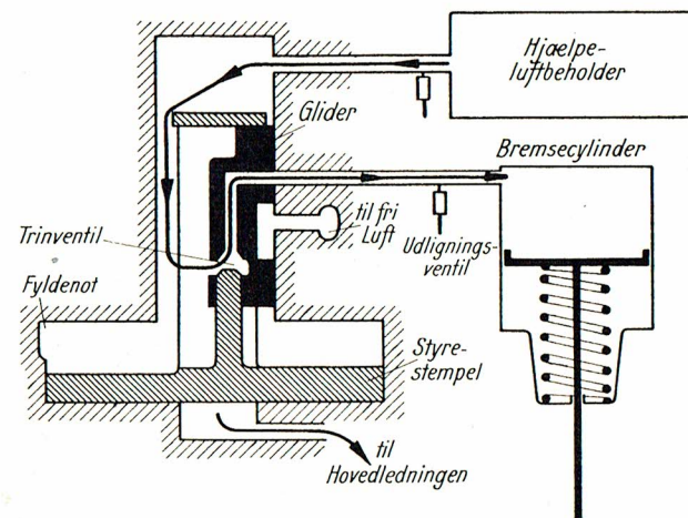
Fig. 55 Bremsstilling
