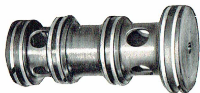
Hovedstyreglider
