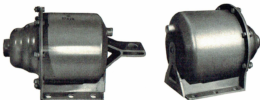
Fig. 63 Staalbremsecylinder med Balancebærer uden Balancebærer
