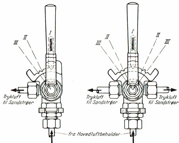
Fig. 72 Sandhanen
