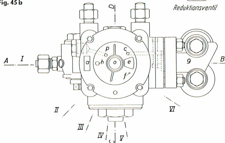
Fig. 45 a—c Snit af Drejeglides-Førerbremseventil Nr. 8
