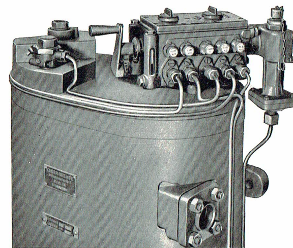
Fig. 33 Pumpehoved med Smørepumpe KL5 og Smørepumpedrevet
