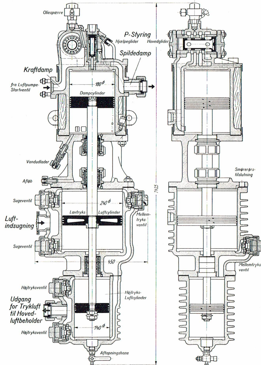
Fig. 7 Snit af Totrins-Luftpumpe med P-Styring
