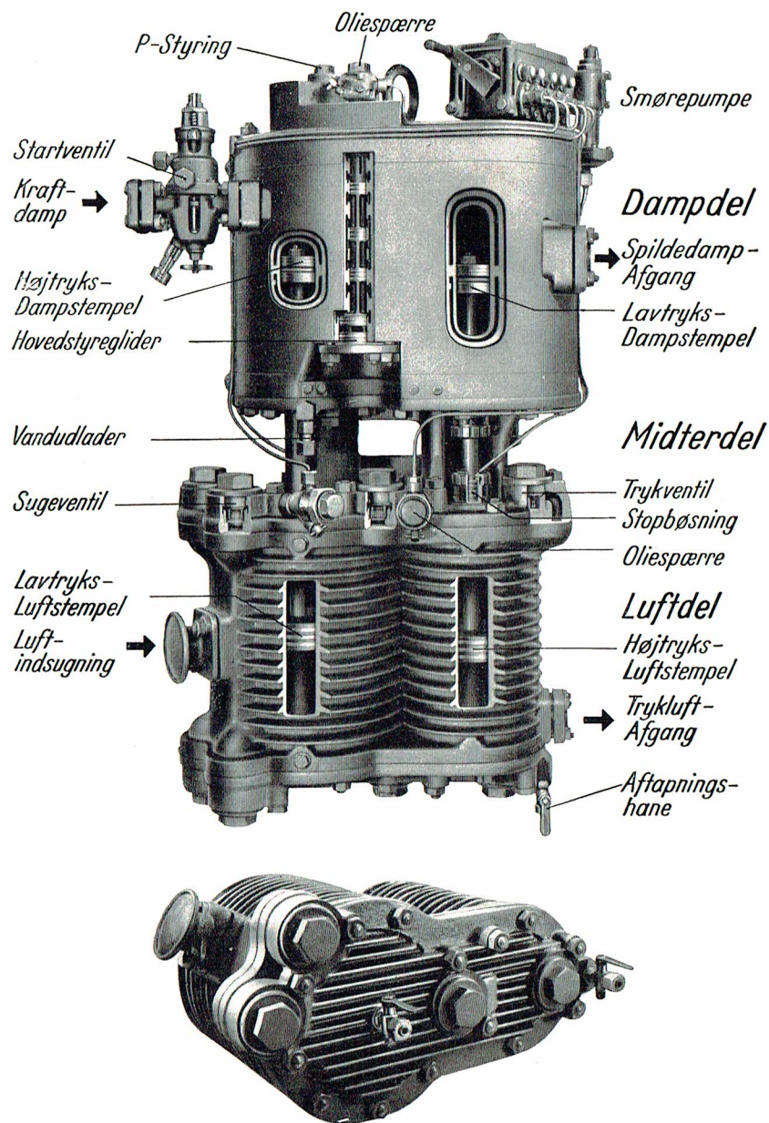
Fig. 14 Udsnit i Dobbelt-Compound-Luftpumpe med P-Styring
