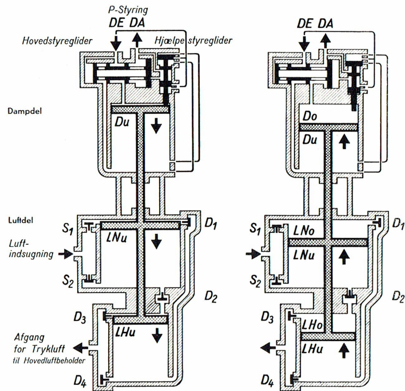
Fig. 8 Totrins-Luftpumpens Virkemaade
