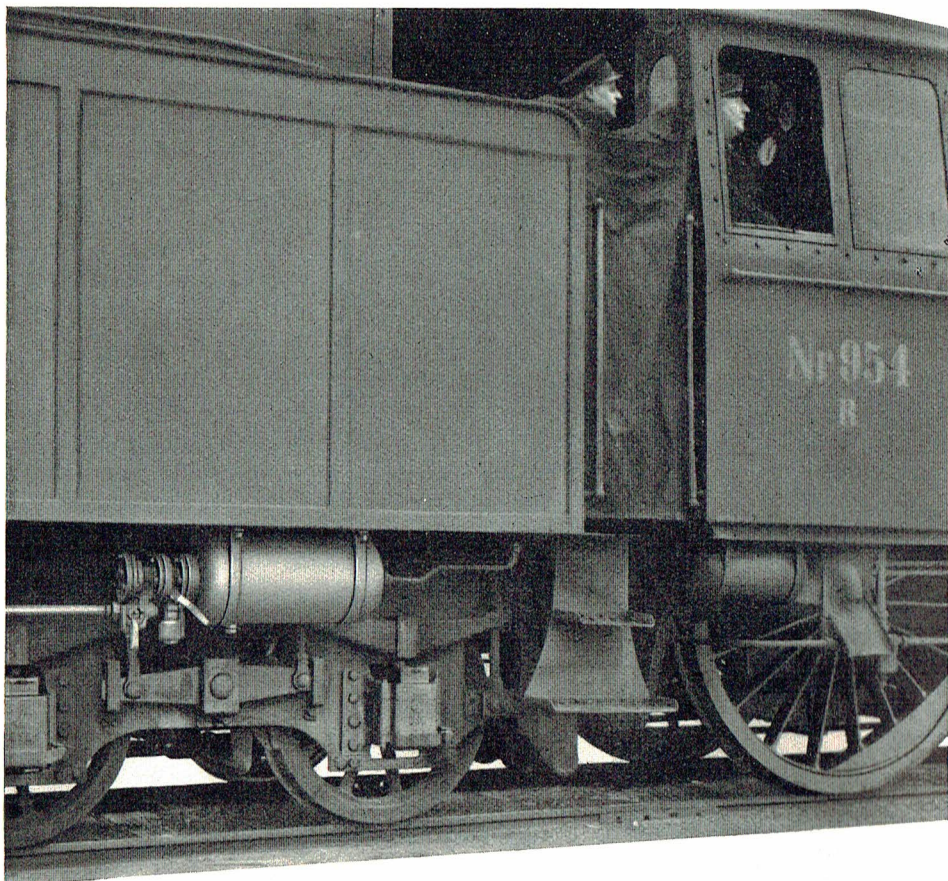
Fig. 75 K1-Styreventil, GP-Ventil og Hjelpeluftbeholder paa Tenderen til Lokomotiv Litra R
