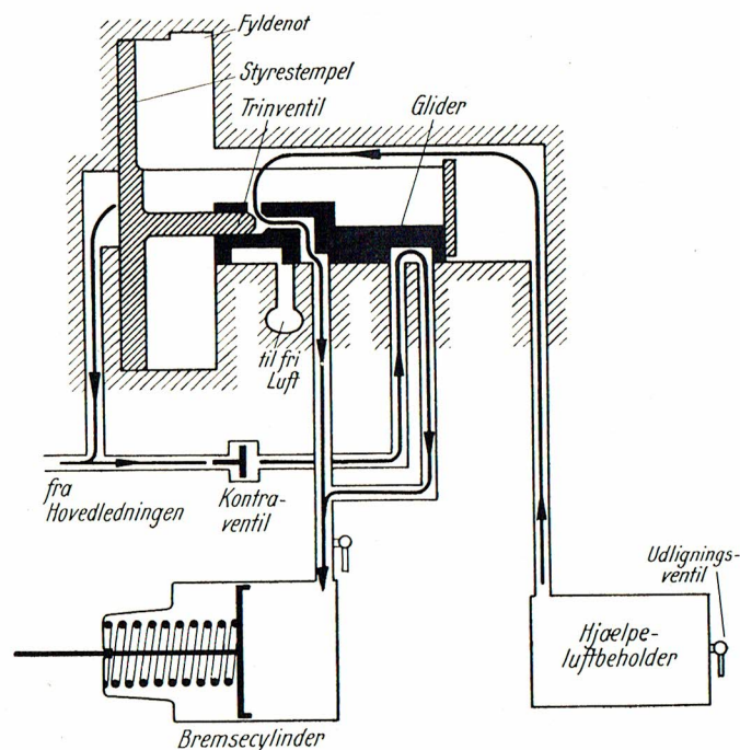
Fig. 81 Farebremsstilling
