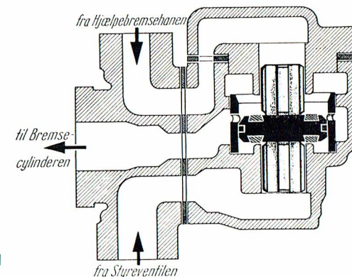
Fig. 89 Dobbeltkontraventil
