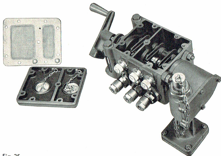
Fig. 25 Smørepumpe KL3 for tre Smøresteder, med affaget Dækslet
