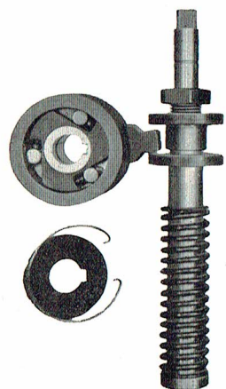
Trykstempel med Gaffelende, Tilbagetryksfjeder og Skraldefriløb
