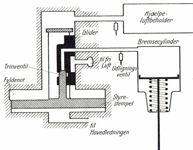
Fig. 56 Bremseafslutningsstilling
