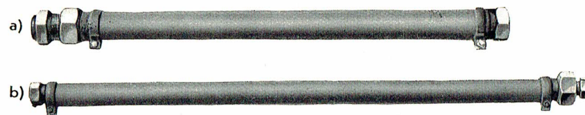
Fig. 69 Slangeforbindelser mellem Lokomotiv og Tender a) for Hovedledning, b) for Hjælpebremseledning
