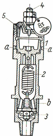
Fig. 41 Snit af Sikkerhedsventil AKL
