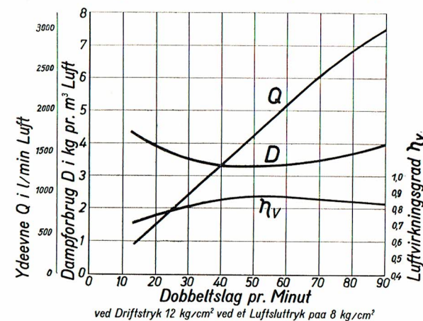
Fig. 13 Dampforbrug, Præstation og Luftvirkningsgrad for Dobbelt-Com- pound-Luftpumpen ved Drifttryk 12 kg/cm 2 ved et Luftsuttryk paa 8 kg/cm 2
