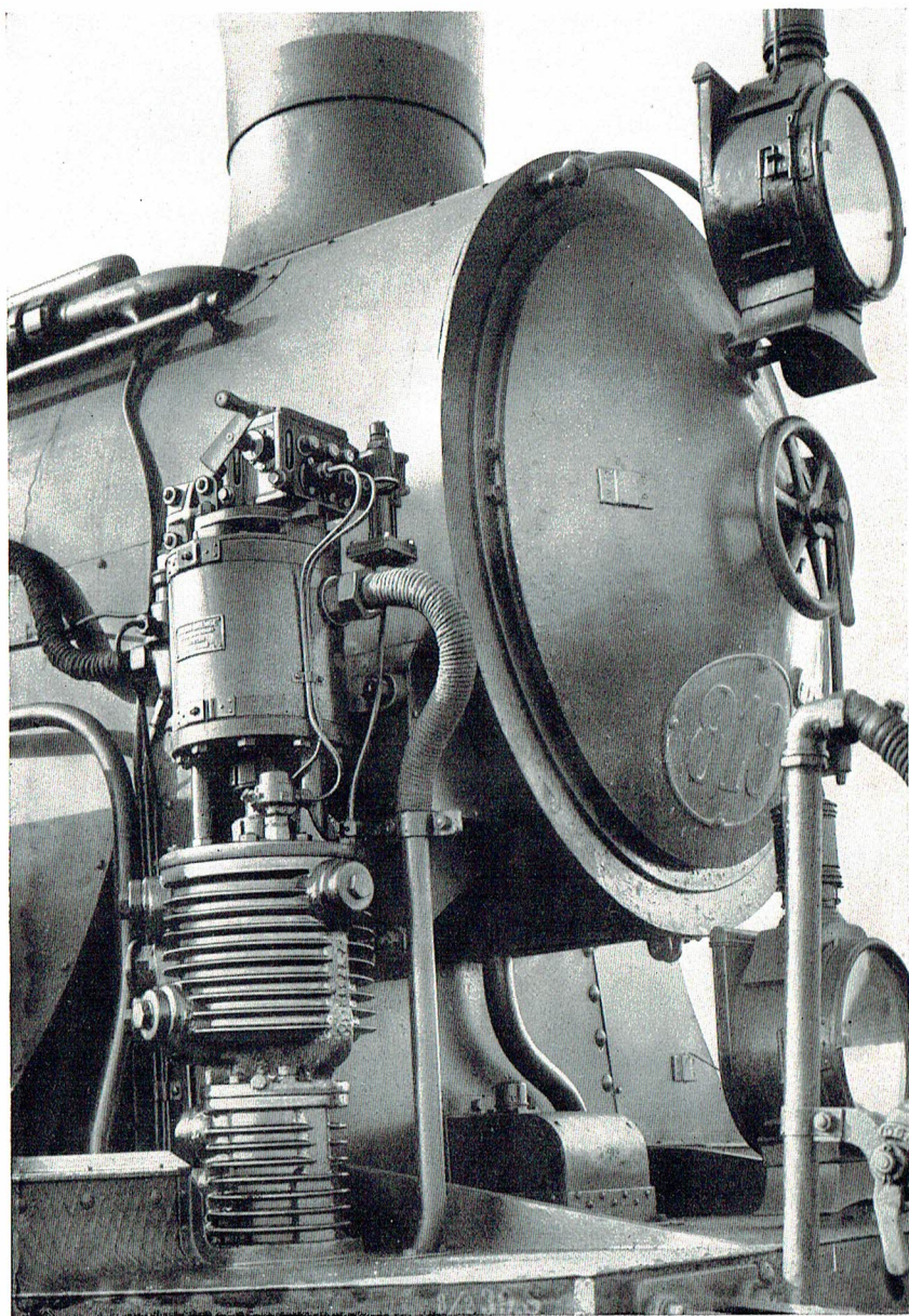
Fig. 4 Totrins-Luftpumpe med P-Styring og luftdrevet Smørepumpe KL3 paa et dansk Godstogslokomotiv Liira D
