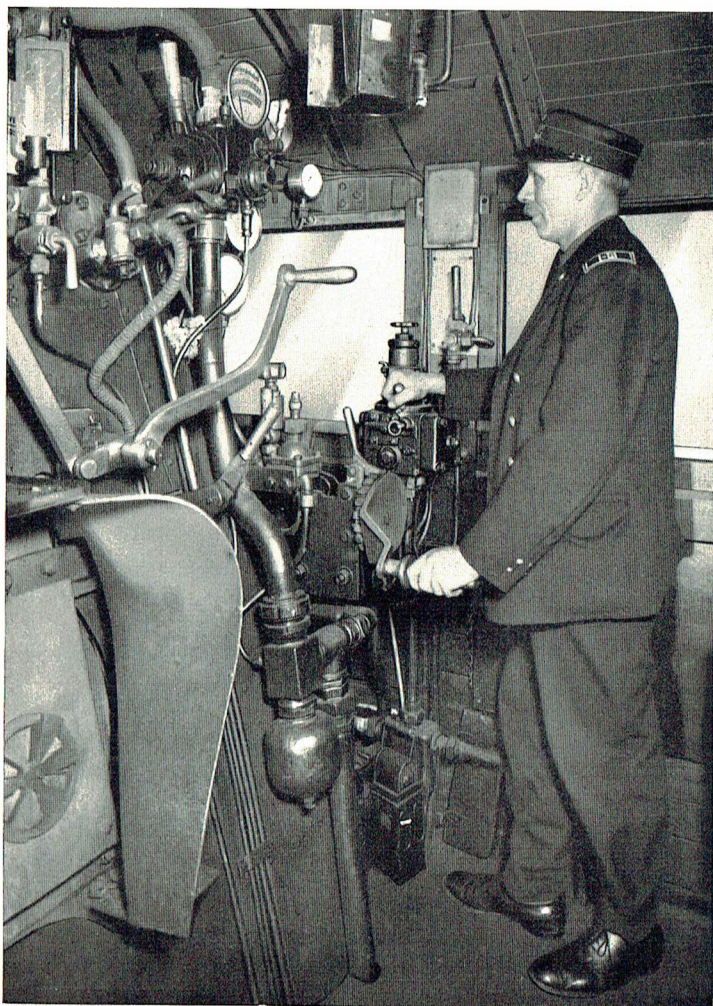
Fig. 48 Automatisk Førerventil, Konstruktion Knorr, i Førerhuset paa et dansk Lokomotiv
