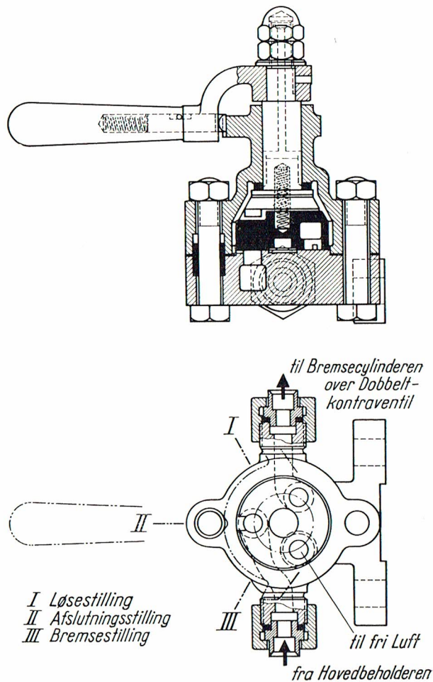
Fig. 87 Snit af Hjælpebremsehane
