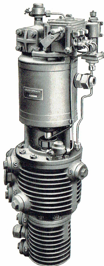
Fig. 26 Totrins-Luftpumpe med Smørepumpe KL 3 for tre Smøresteder
