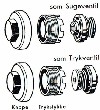
Fig. 12 Indbygning af en Pladeventil
