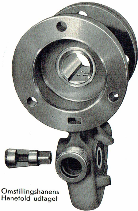
Fig. 77 Gliderspejlet i K1-Styreventilhuset
