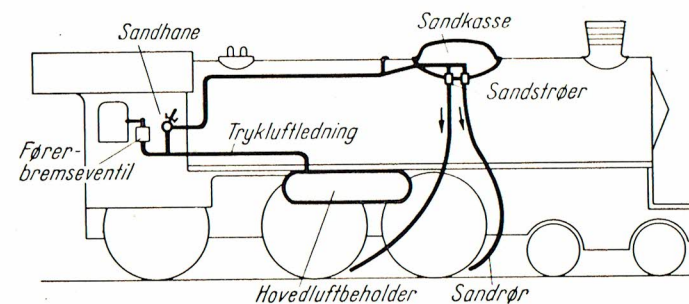
Fig. 73 Arrangement af Sandstrøpparatene paa et Lokomotiv Litra R
