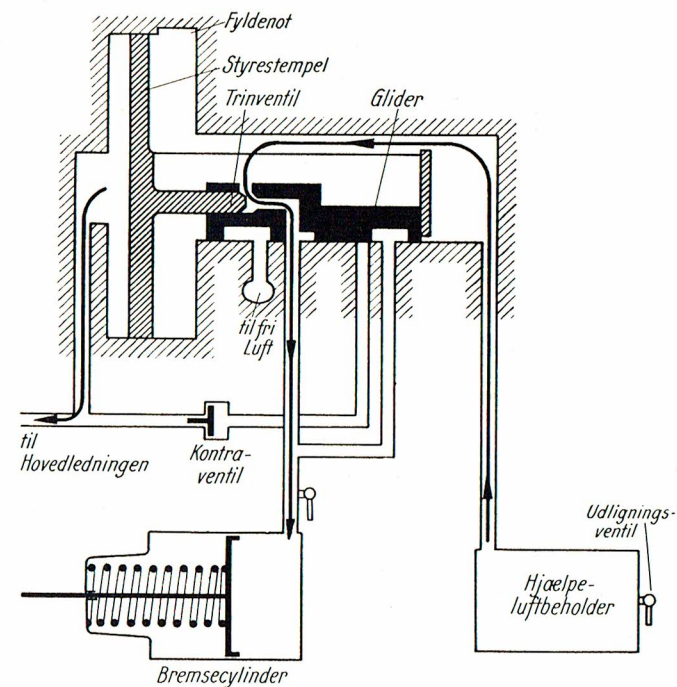
Fig. 80 Driftsbremsestilling
