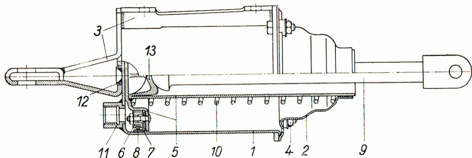
Fig. 62 Staalbremsecylinder samlet
