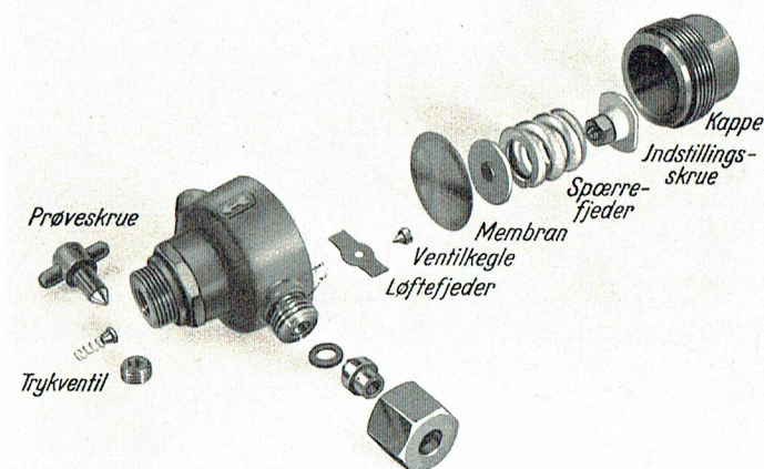
Fig. 39 Enkeltdele til Knorr Oliespærre
