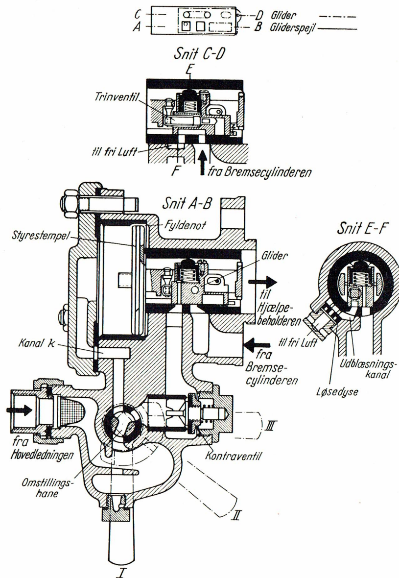
Fig. 82 Snit af K1-Styreventil i Løsestillingen
