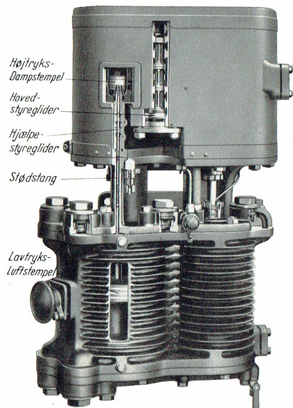
Fig. 21 Snit i Dobbelt-Compound-Luftpumpe med Nielebock-Styring
