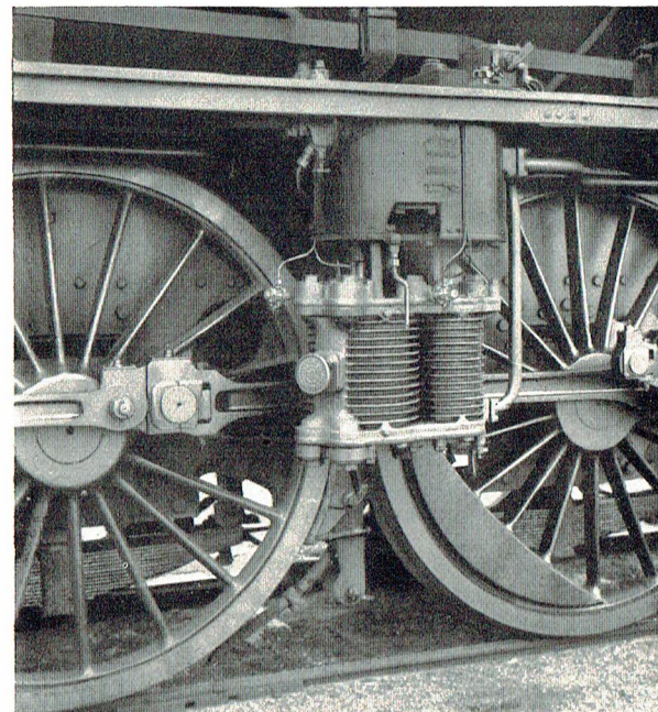
Fig. 20 Dobbelt-Compound-Luftpumpe paa et dansk Persontogslokomotiv Litra R
