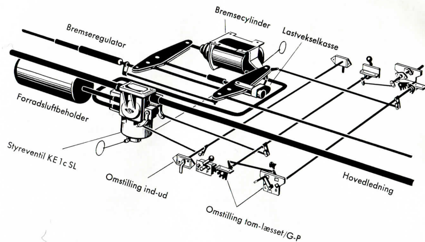
Fig. 28. S-mærket godsvogn med Knorr-godstogs-personotogsbremse KE
