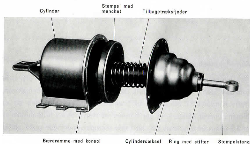
Fig. 15. Stålbremsecylinderens enkeltdele
