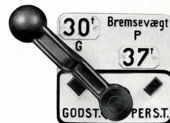
Fig. 19. Omstilling godst. — pers.t.
