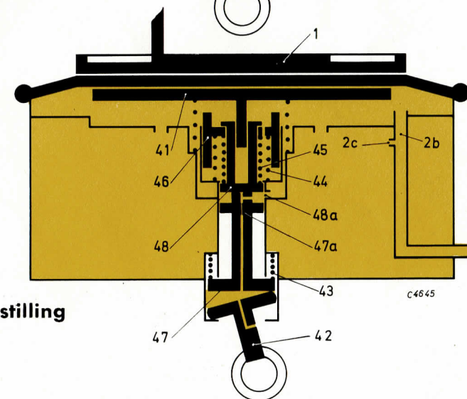
Fig. 3: Bremse (afslutnings) stilling (mindre tryk i hovedledning end i styrekammer A)
