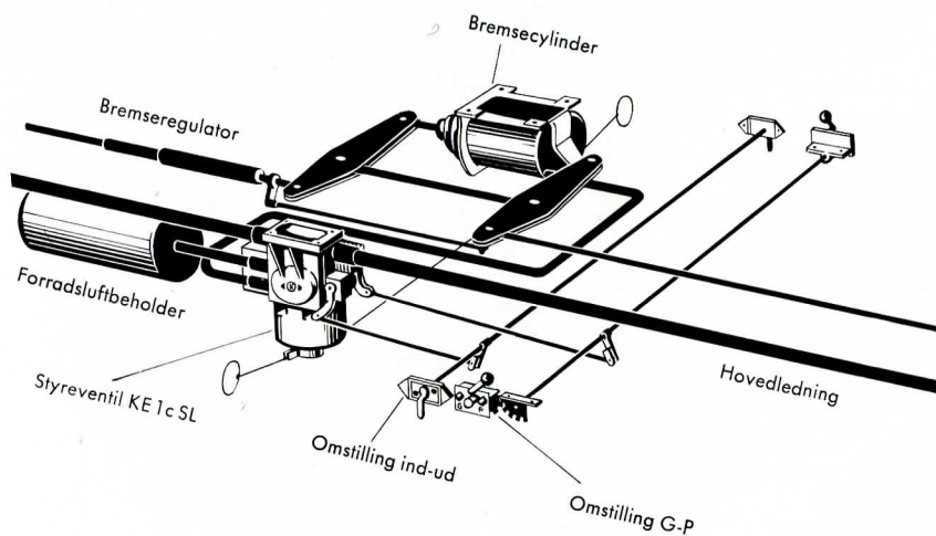
Fig. 29. Personvogn med Knorr-personotogsbremse KE.
