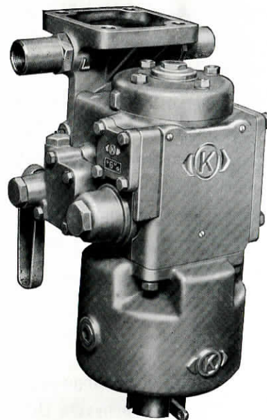
Fig. 10. Styrekammer A monteret på enheds-grundventilen
