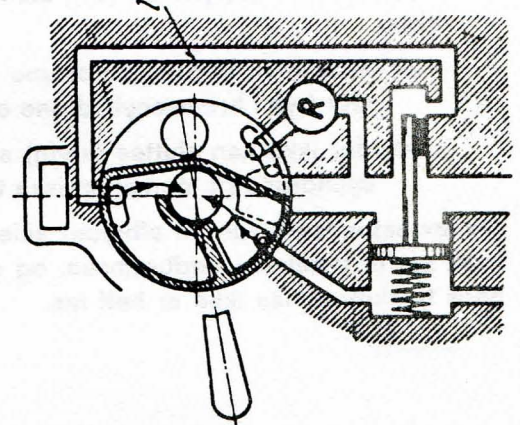
Stilling V: Driftsbremsestilling
