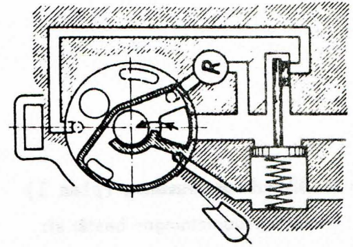
Stilling VI: Førebremsestilling
