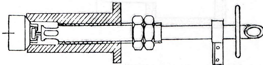
Fig 2. Brandventil (skematisk).
