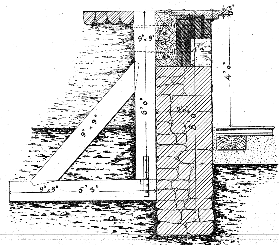
Snit a-b.
