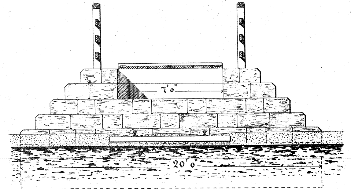
Længdesnit.
