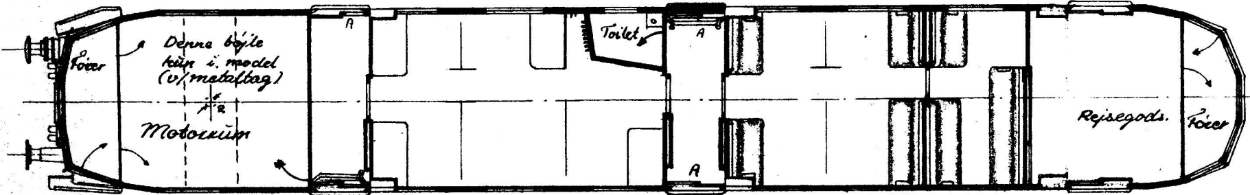
Snitbillede af vognkassen. Vogngaule er ens, men spjældte. Dørdetaljer mækt. "A" er ens.
