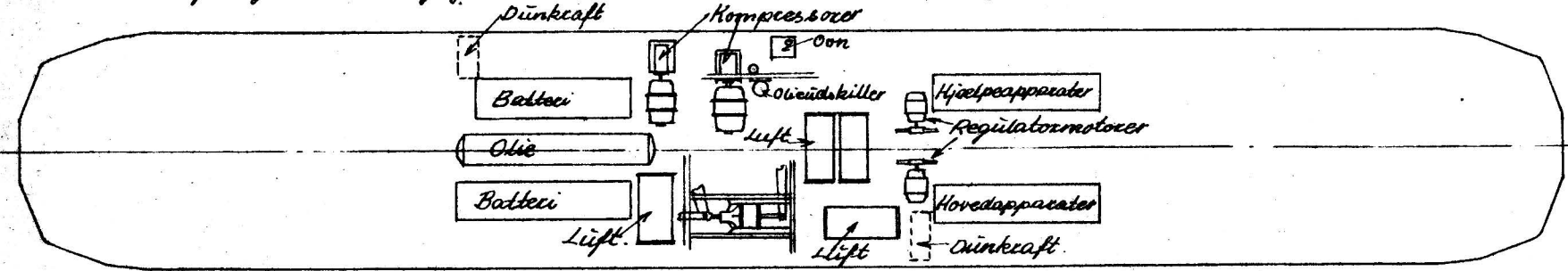
Undervogn med detaljer (bremsedetaljer udeladt) samt disses anbringelser set ovenfra.
