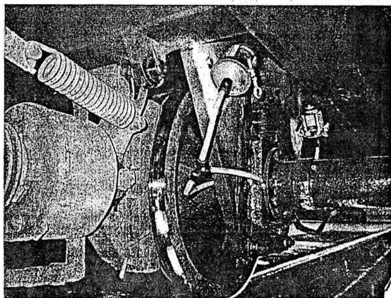
Smøring af kulissestyr
