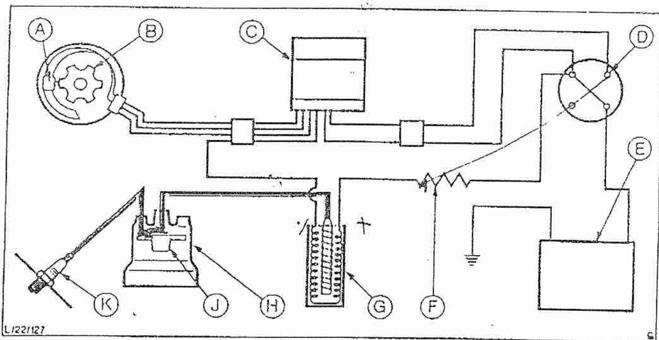
Fig. 19 - Kontaktløs tændingssystem skematisk (strømvejen ved begyndelsen af tændingsimpulsen) A - Strømfordelerens opsamlerspole uden strømgennemgang (skiftetpunkt fra negativ til positiv) E - Batteri H - Strømfordelerdæksel B - Kogestykke direkte modsat opsamlerblokken F - Formodstand J - Rotoren leder højspænding til den pågældende cylinder C - Modulet afbrudt G - Spolens primærkreds afbrudt med resulterende højspænding K - Tændrøret leder D - Tændingskontaktens startmotor-klemme
