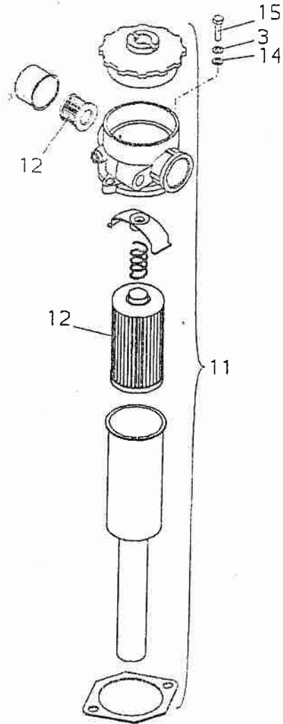
Returfilter
