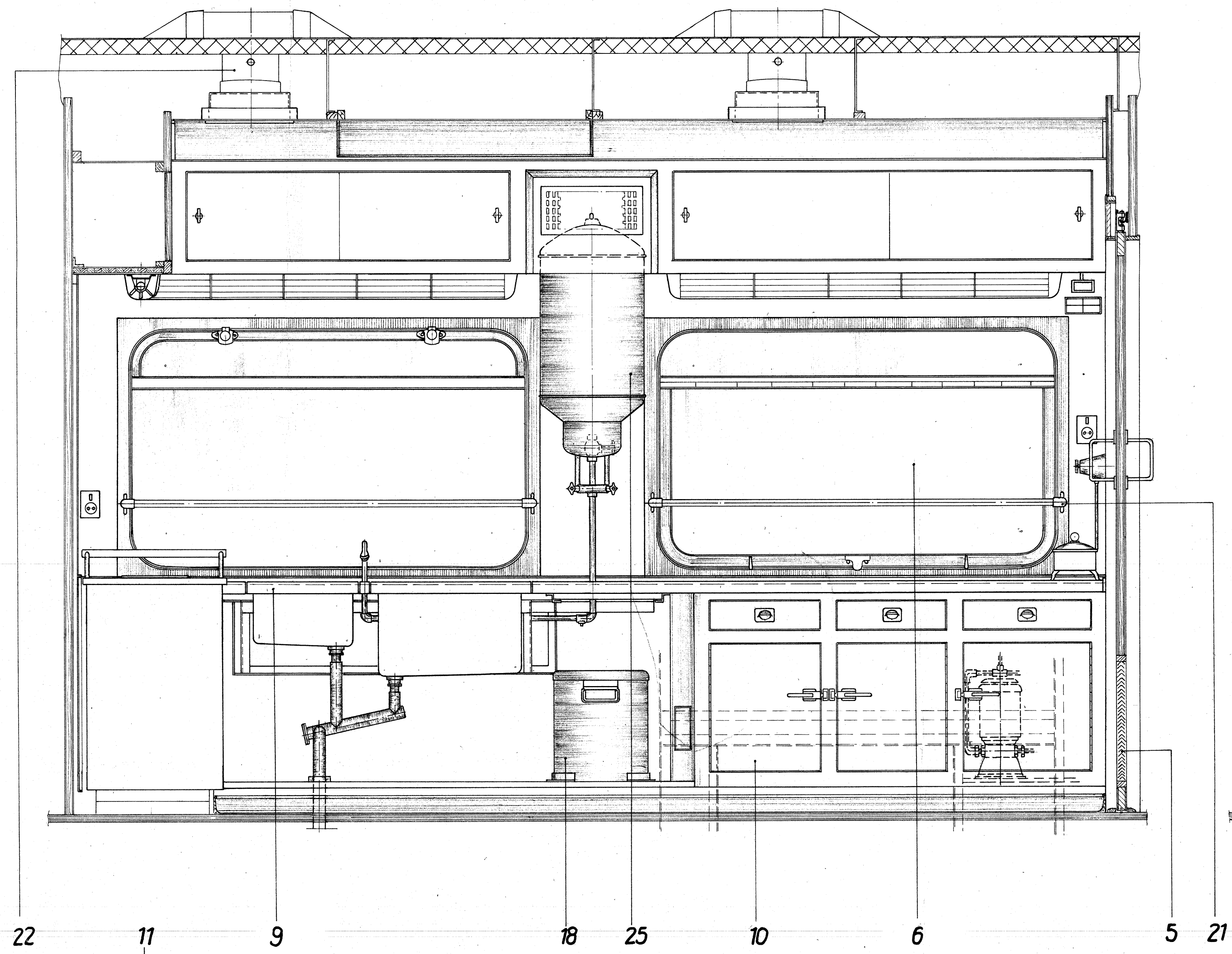
Schnitt A - A
