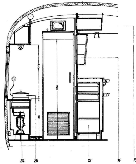
Schnitt C - C
