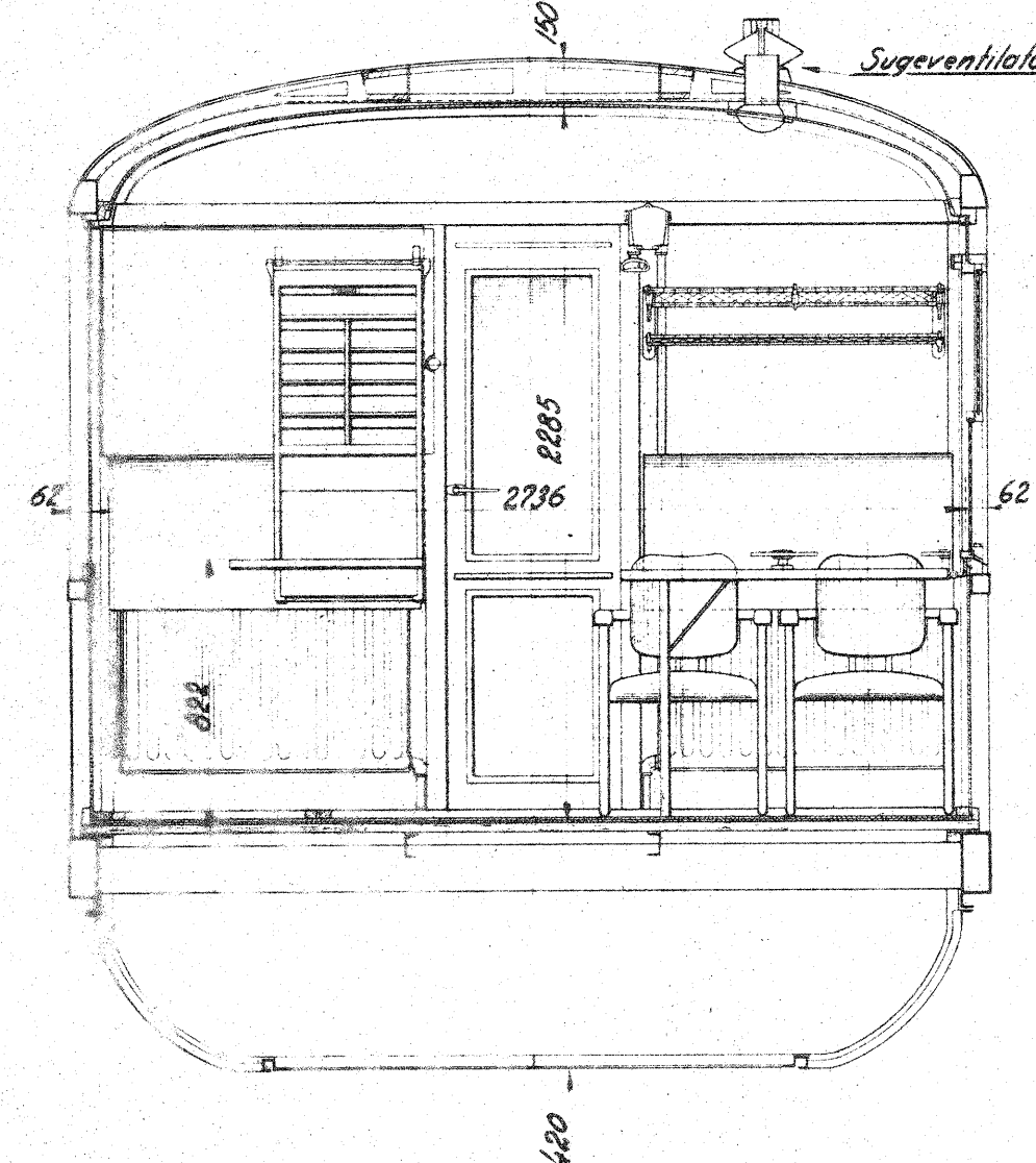
Snit i-k
