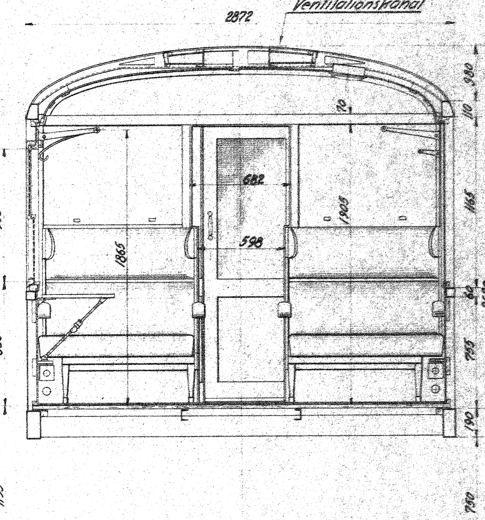
Snit p-q
