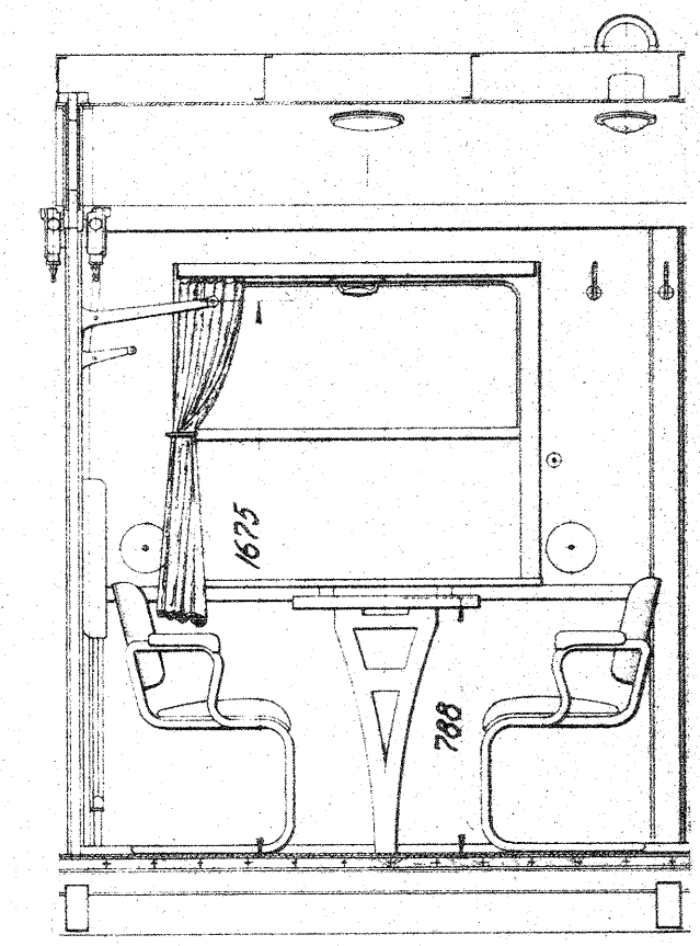
Snit n-o
