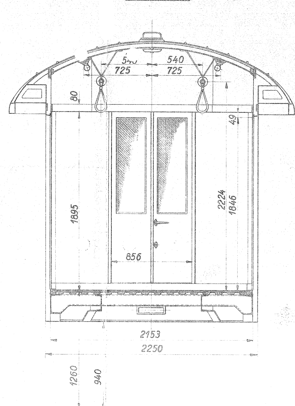
Snit: B-B
