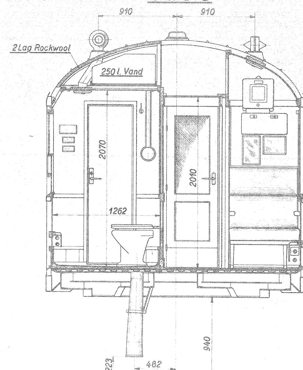
Snit: D-D
