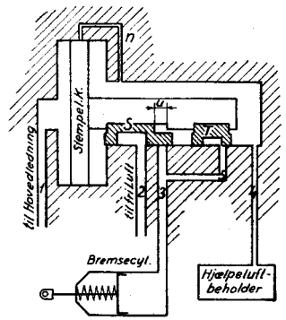
c. Bremseafslutningsstilling.
