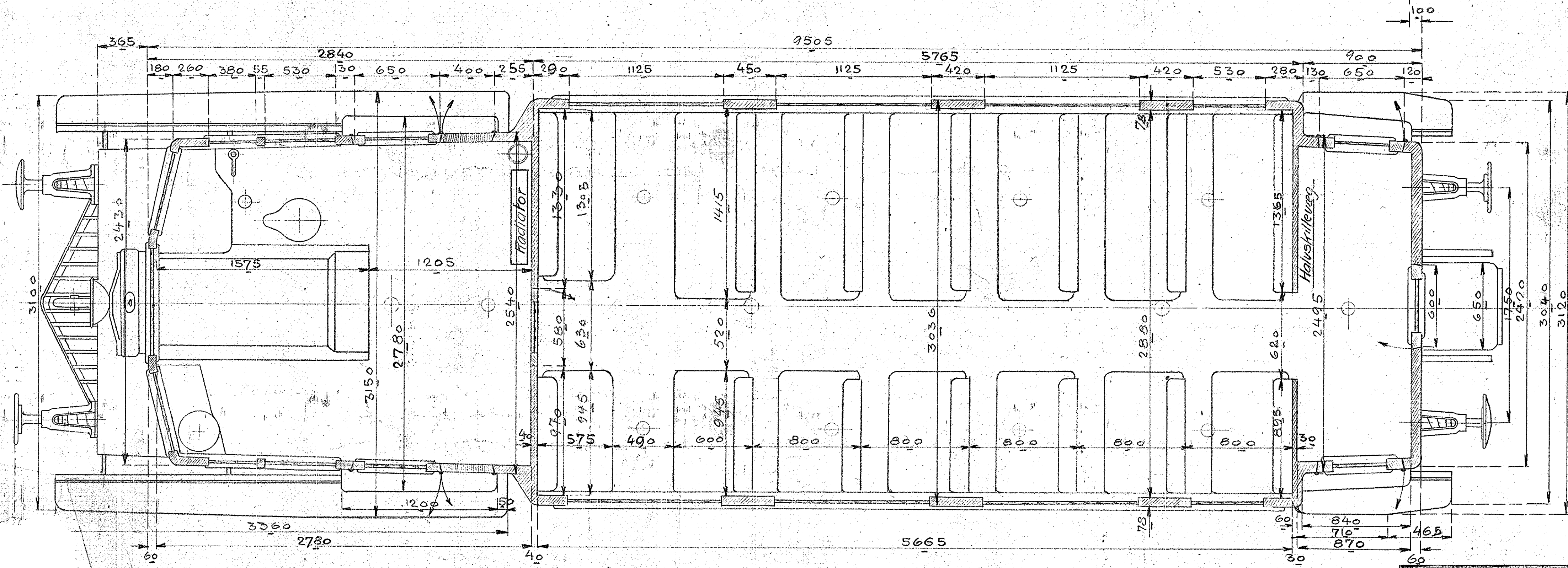
Benzin-mekanisk Motorvogn. Lyngby-Nærum Jernbane - 35 Siddepl. Skala 1:20
