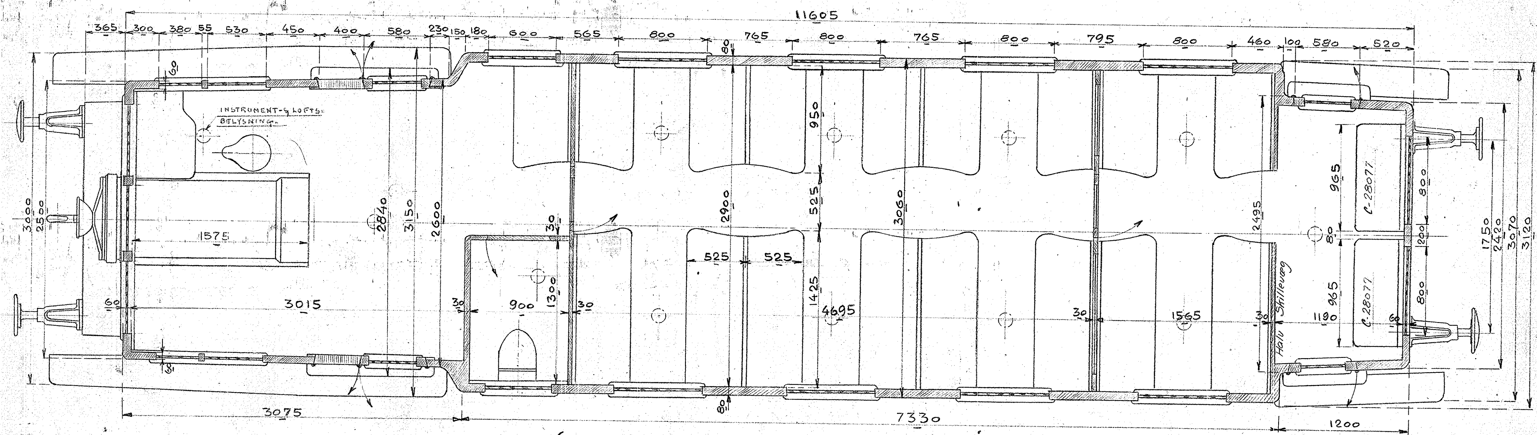
— Hjørring Privatbaner. — Ombygning af Personvogn til Motorvogn Maal 1:20 — 46 Siddepladser. —
