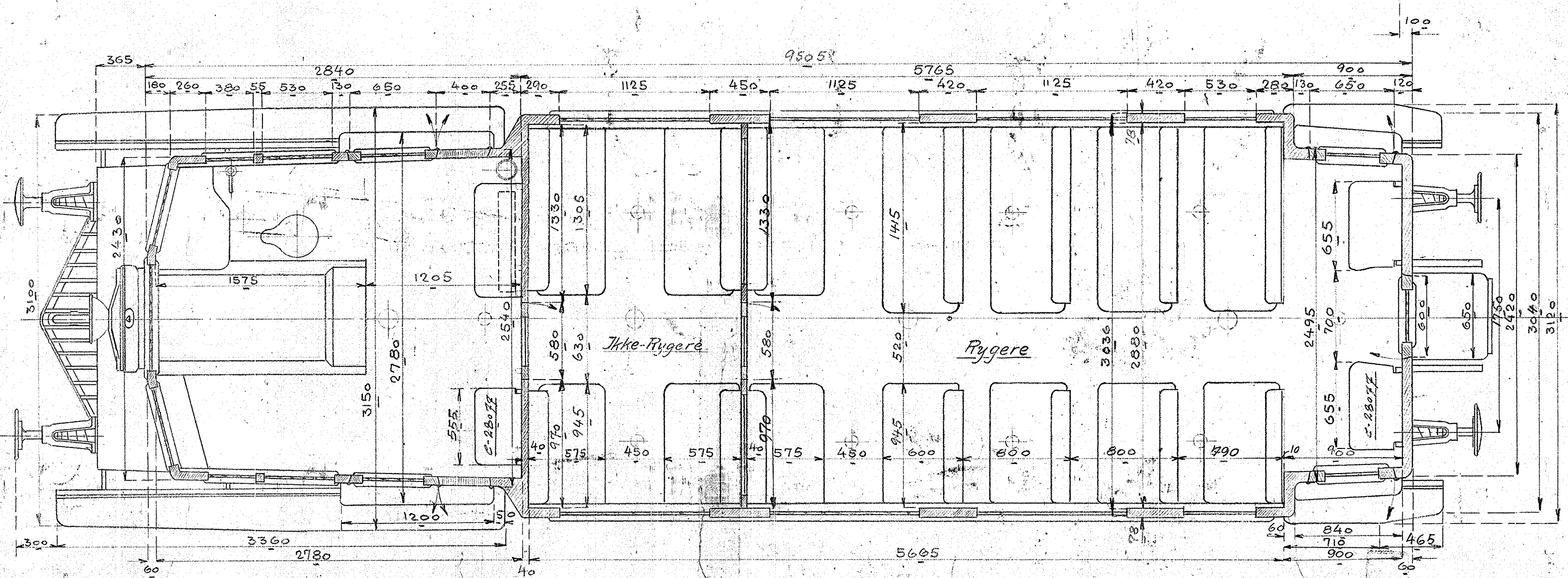
Benzin-mekanisk Motorvogn. Ebeltoft-Trustrup Jernbane-42 Siddepl. Skala 1:20
