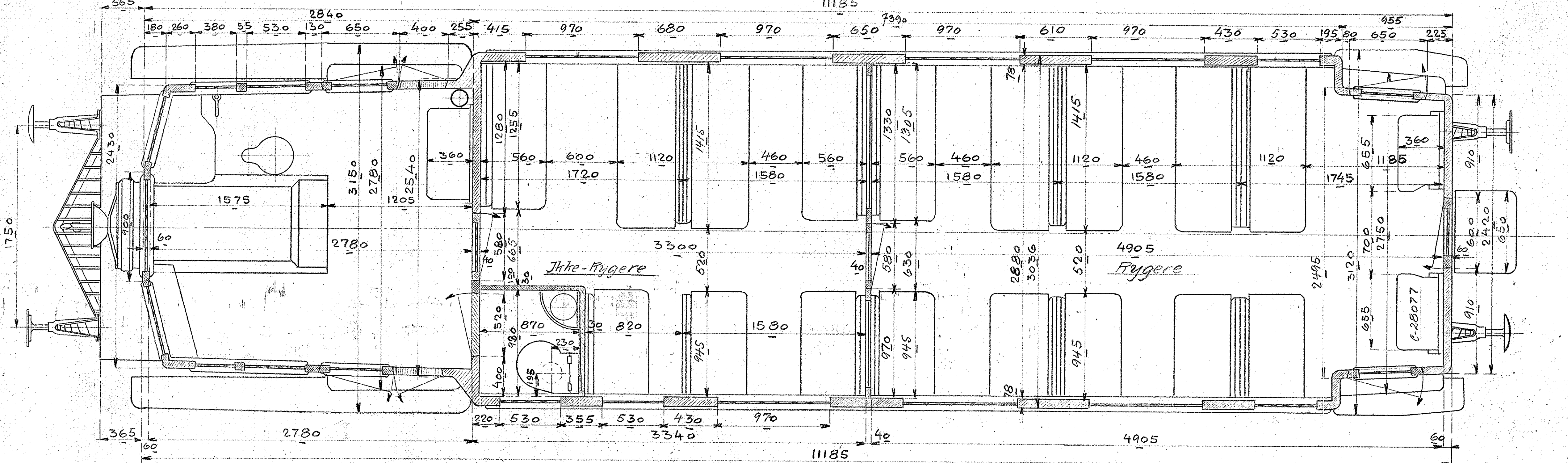
— Thisted-Fjerritslev Jernbane — — Benzin-mekanisk Motorvogn — — 49 Siddepladser — Skala 1:20
