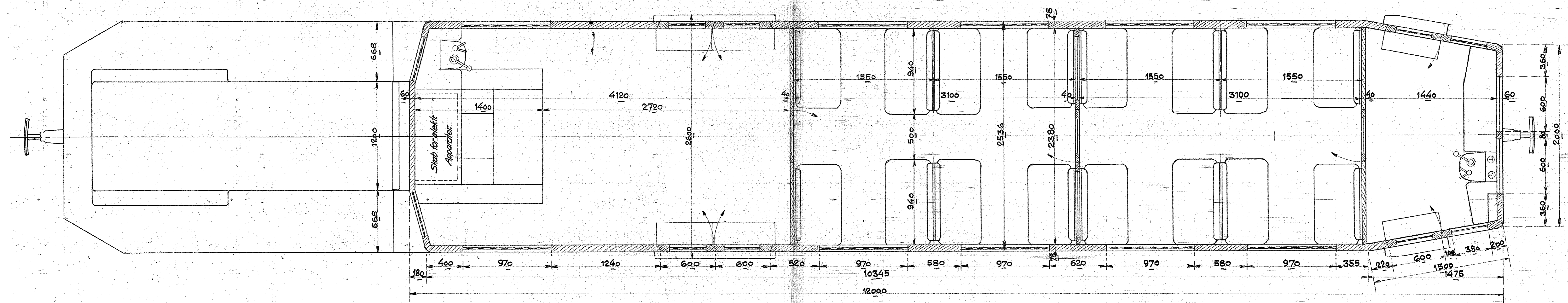
225/250 HK. diesel - elektrisk Motorvogn. Haderslev Amts Jernbaner. 32 Siddepladser. Skala 1:20.
