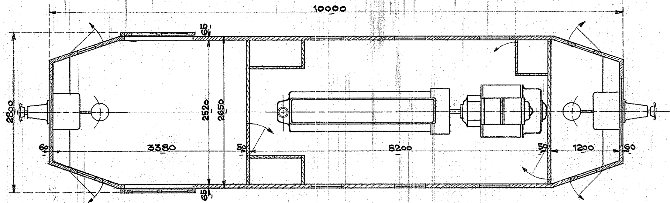
330/350 HK diesel-elektrisk Lokomotiv. 1000 mm. Sporvidde. Skala 1:40.
