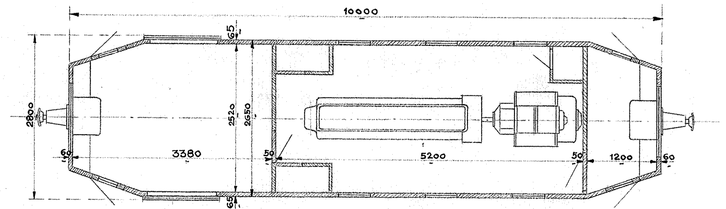
400HK diesel-elektrisk Lokomotiv. 1000mm Sporvidde Skala 1:40.
