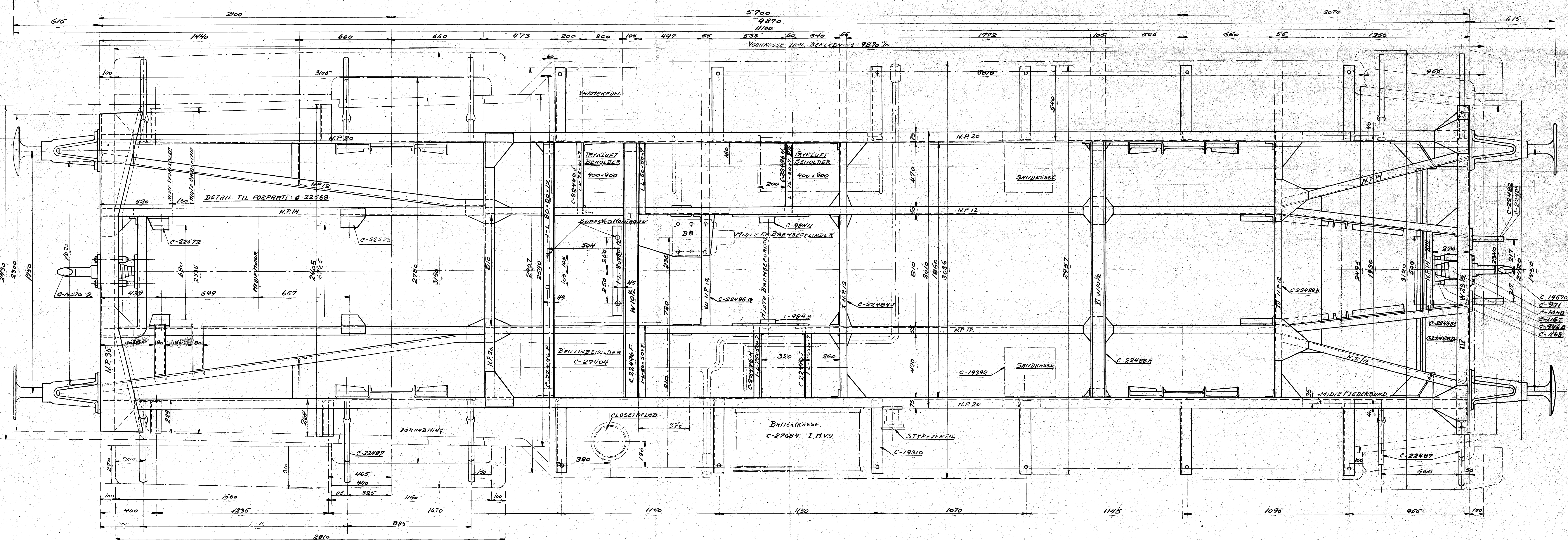
MONTAGETEGNING FOR MOTORVOGN. HONG - TOLLØSE - JERNB. SKALA 1:10
