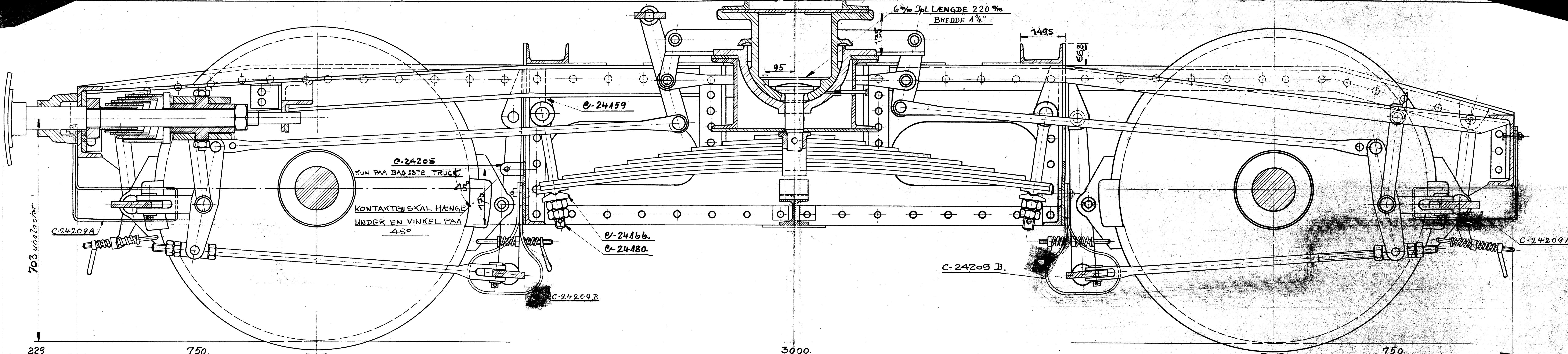
TEGNET FOR UBELASTET VOGN.
