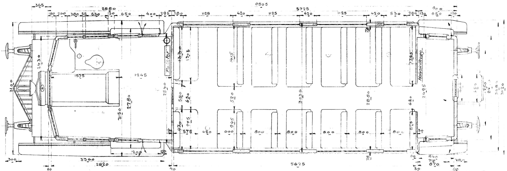
Benzin-mekanisk Motorvogn. Lyngby-Nærum Jernbane - 35 Siddepl. Skala 1:20
