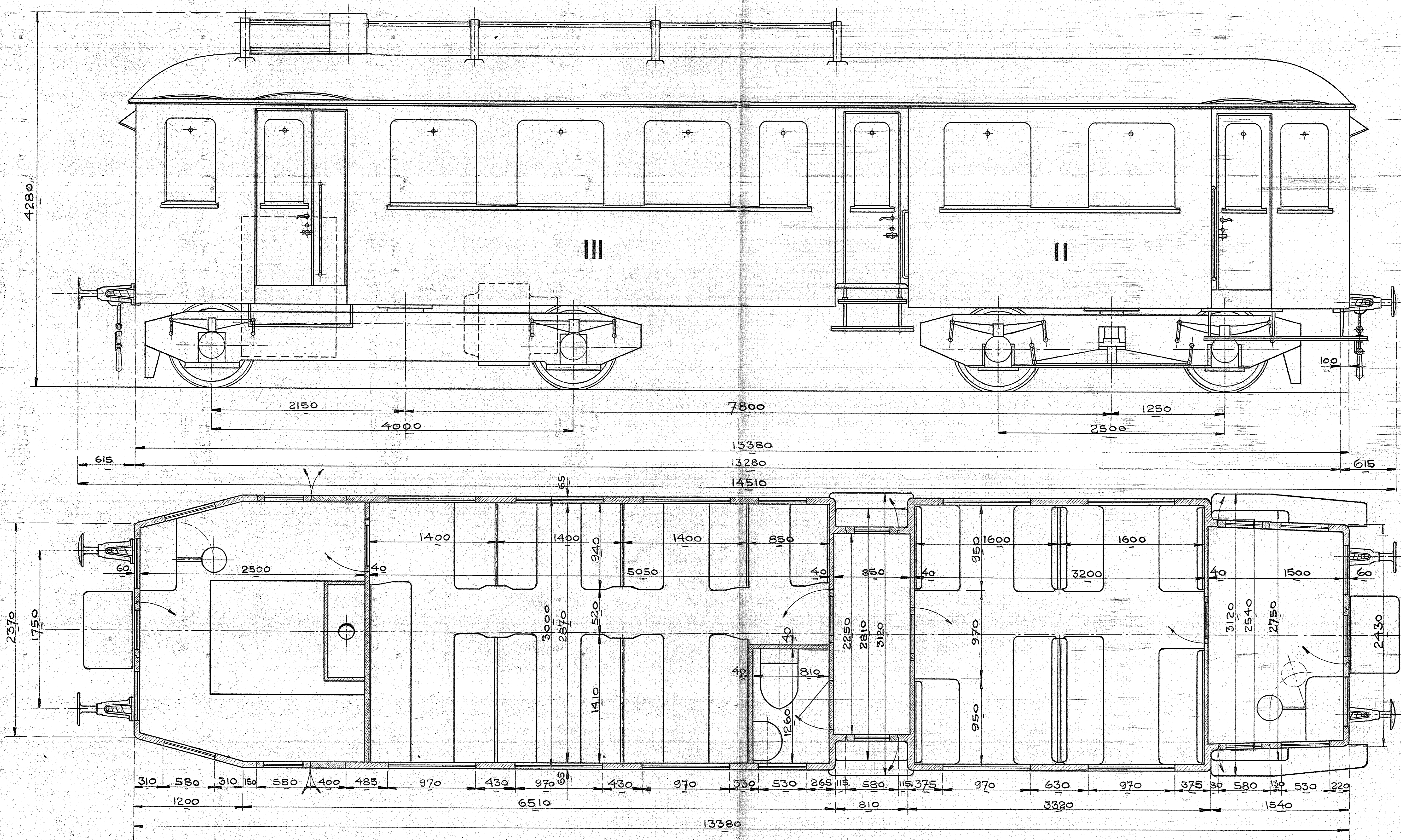
— 120/130 P.S. DIESEL-ELEKTRISCHER TRIEBWAGEN. — — 50 SITZPLÄTZE — SPURWEITE 1435 M M SKALA 1:20
