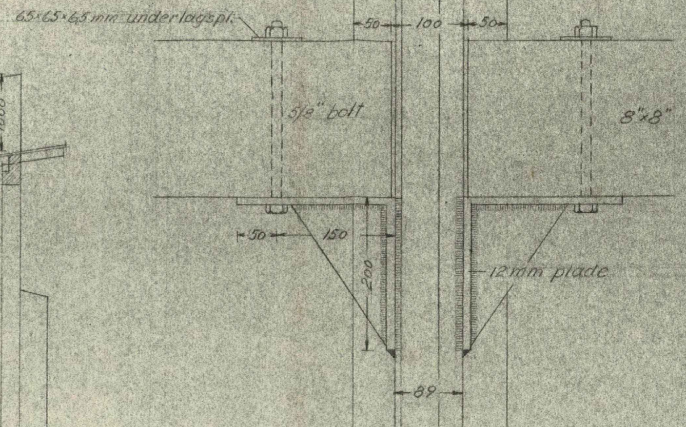
Understøtning af dragere
