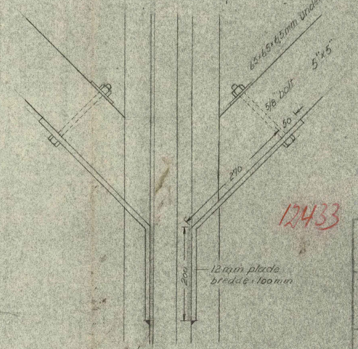
Understøtning af skraabaand
