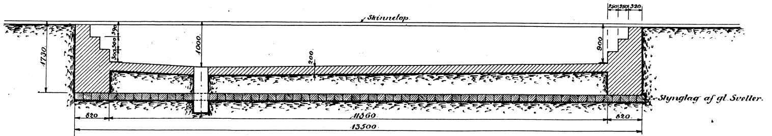
Tværsnit.
