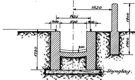
Tværsnit.
