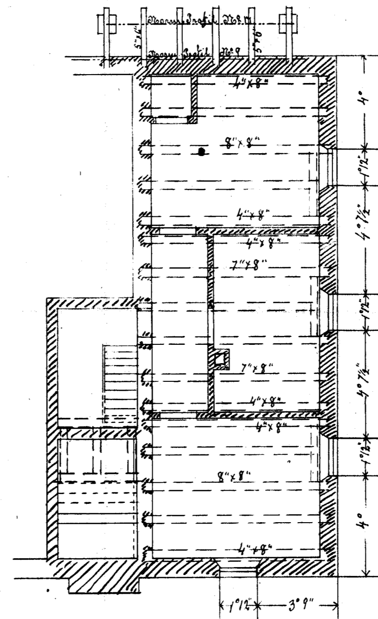
Kælderplan.
