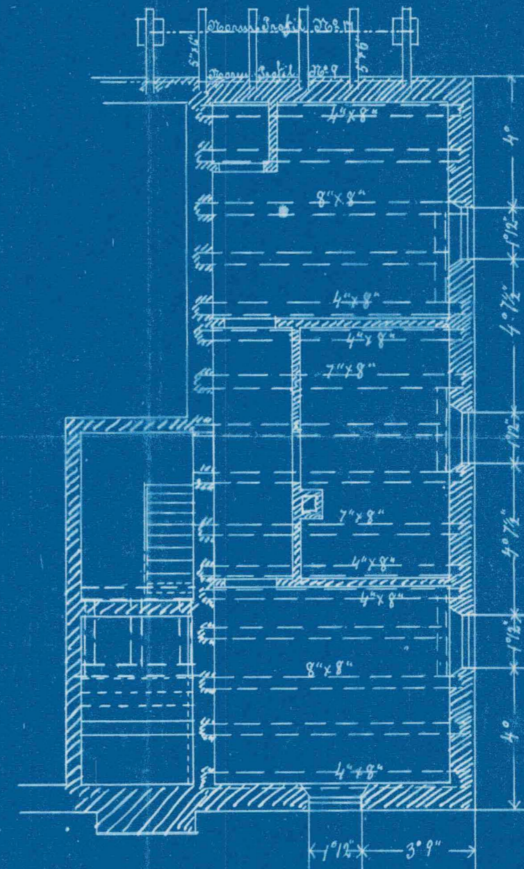
Kalderrplan.
