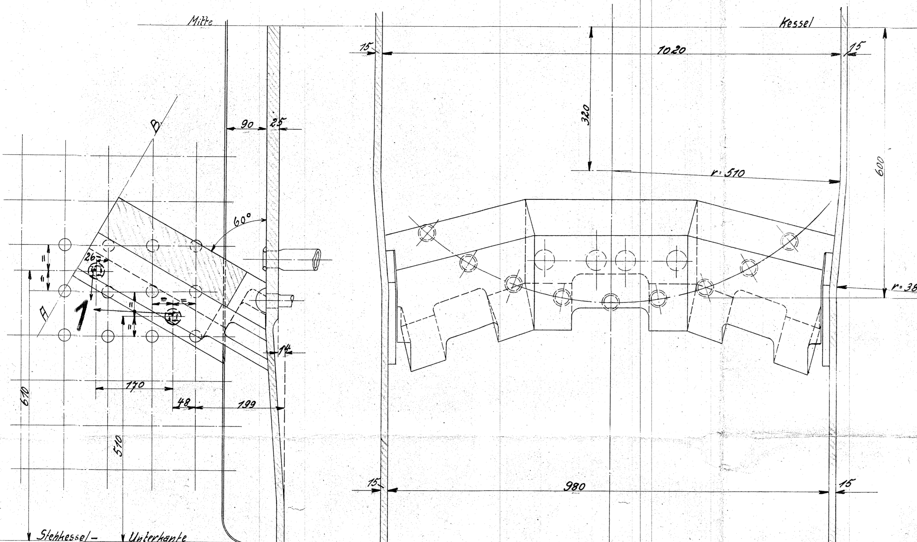
Schnitt A-B
