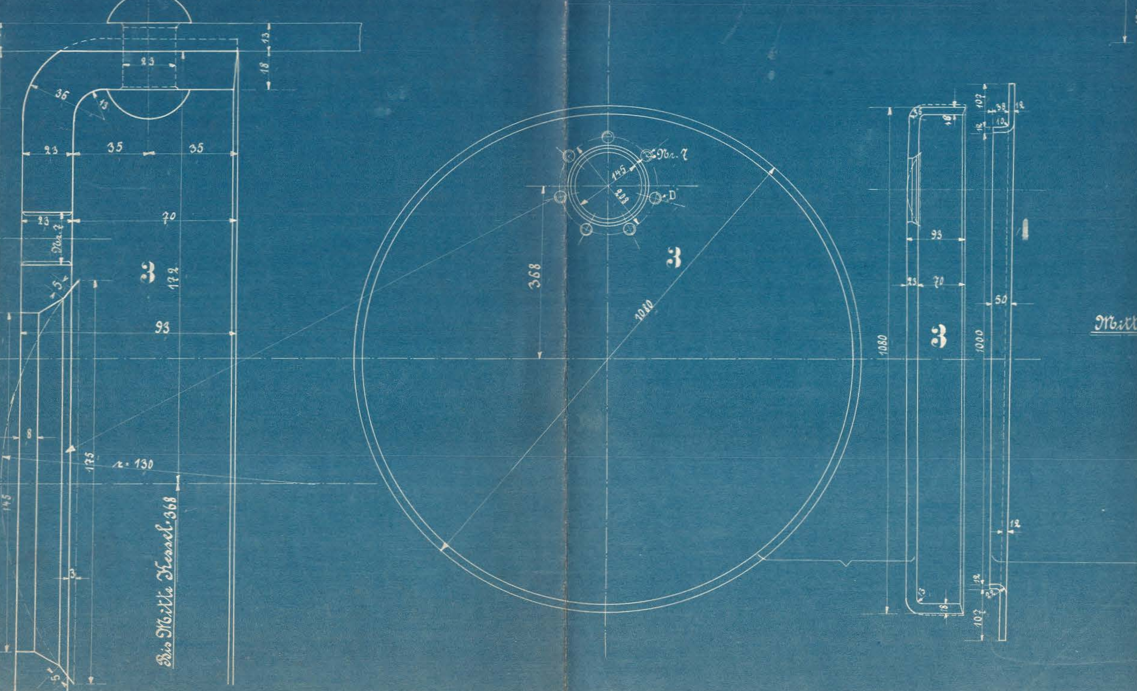
Schnitt durch die Baukammer rohrwand in natürl. Größe
