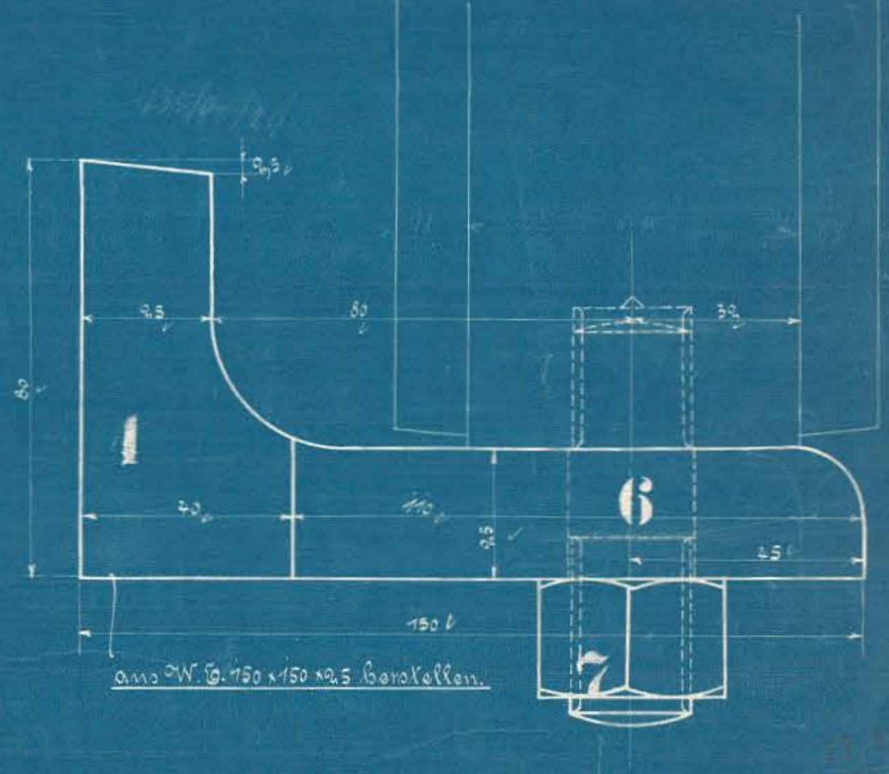
Schnitt C-D
