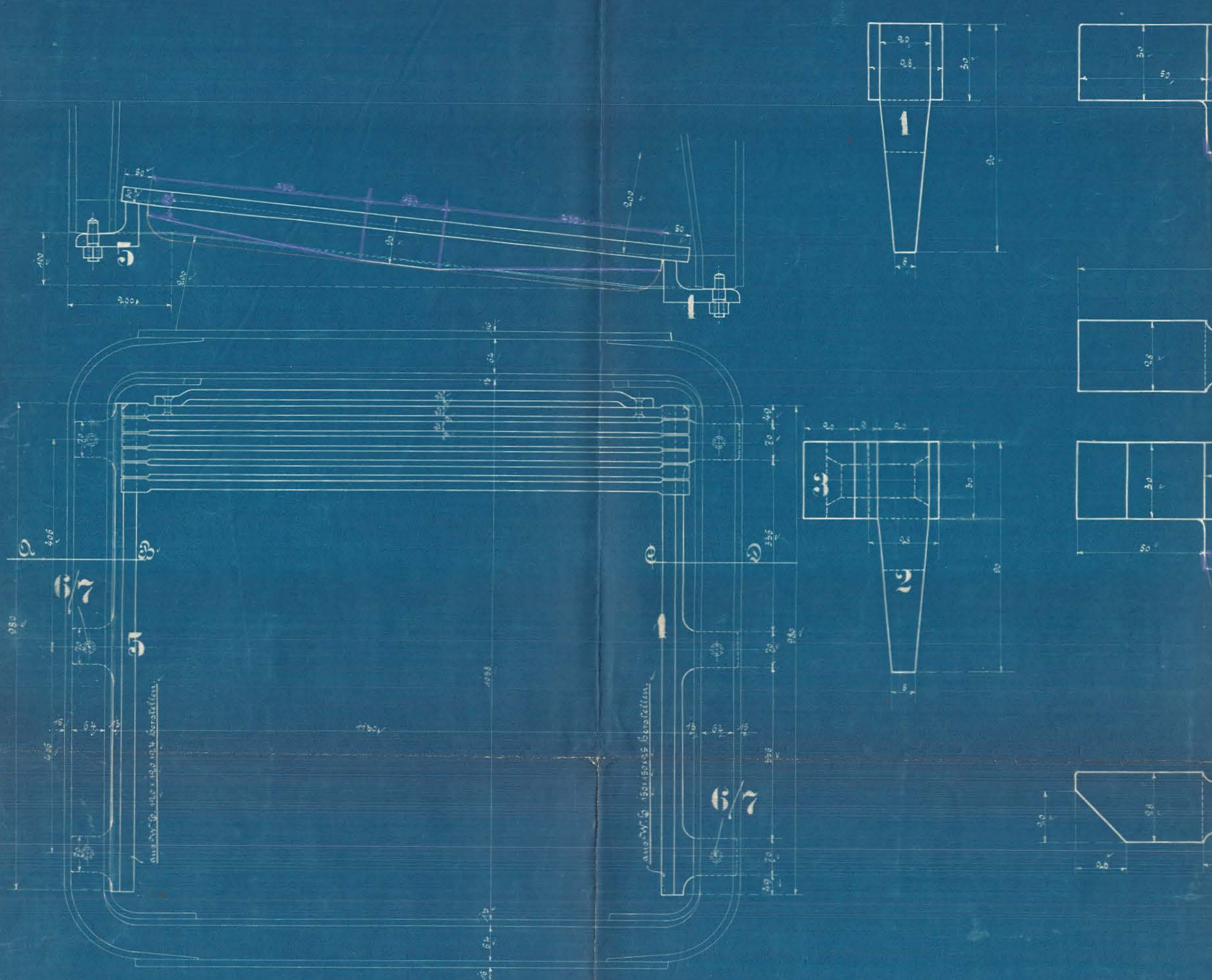
Schnitt A-B
