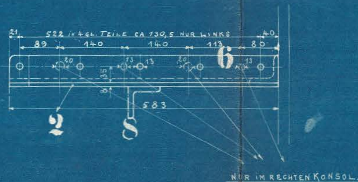
Linke KONSOLE VON HINTEN GESEHEN.
