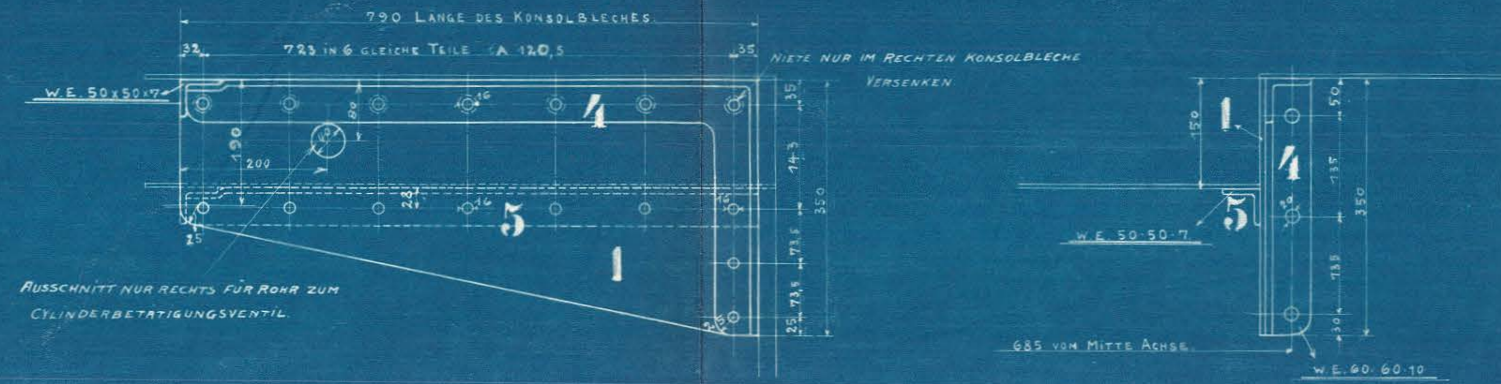
TEILUNG FÜR DIE RECHTE KONSOLE.
