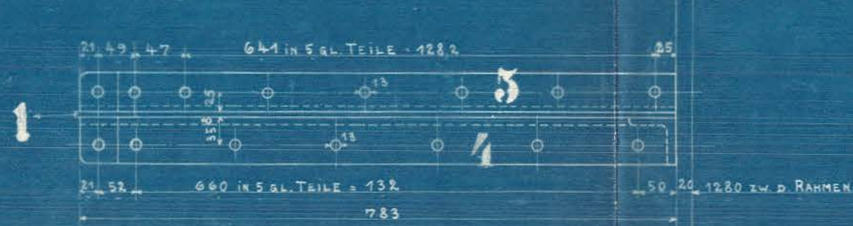
TEILUNG FÜR DIE RECHTE KONSOLE.
