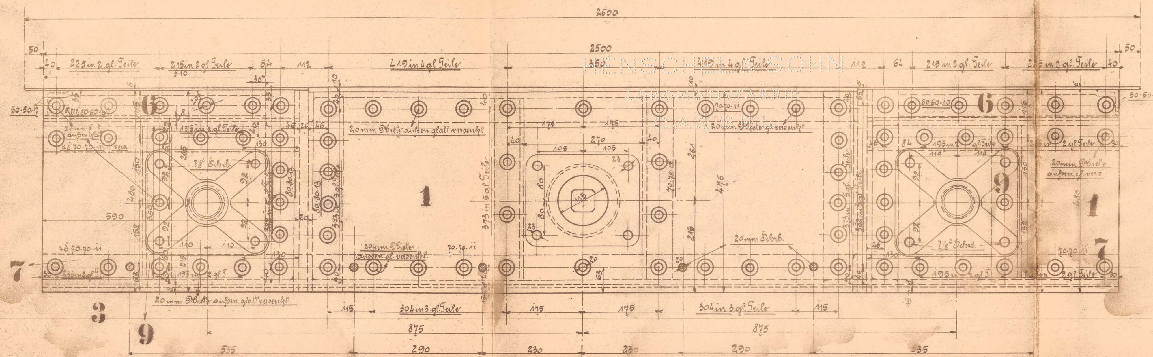
20. Außen 20mm zur Befestigung des Ölbehänges
