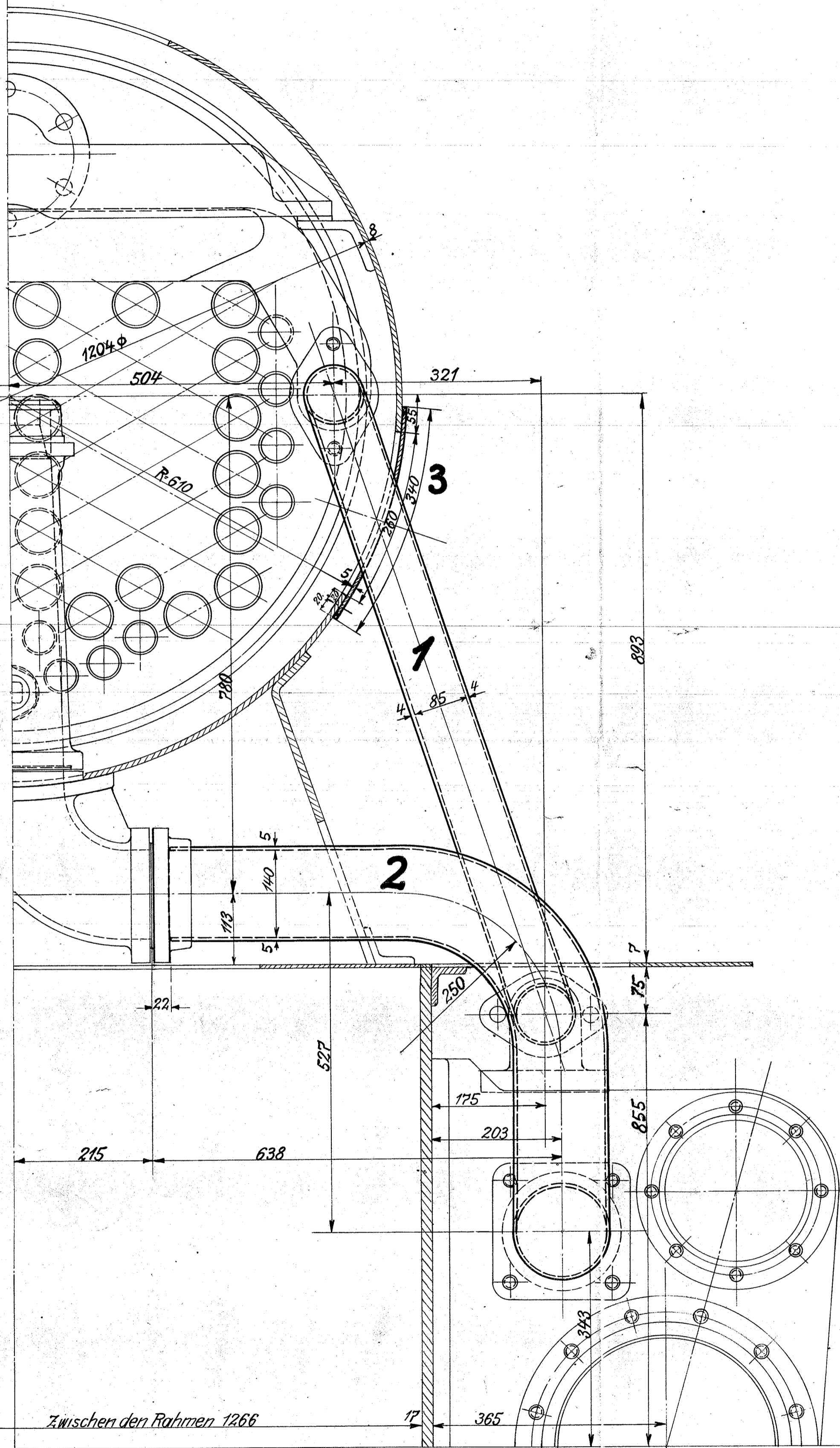
Flansche s. Z. 513.
