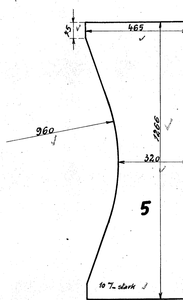
Strebe für hint. Drehgestell
