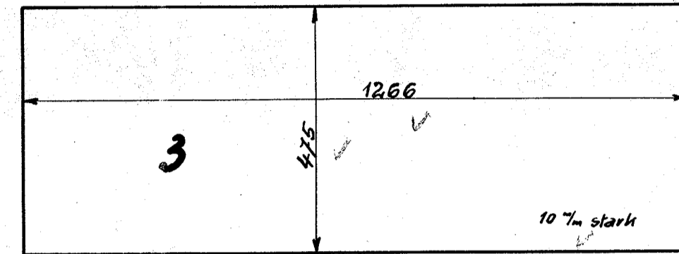
Strebe zw. Laufachse u. Feuerkasten für Bremszylinder
