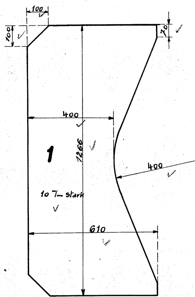
Strebe für hintere Bufferbohle
