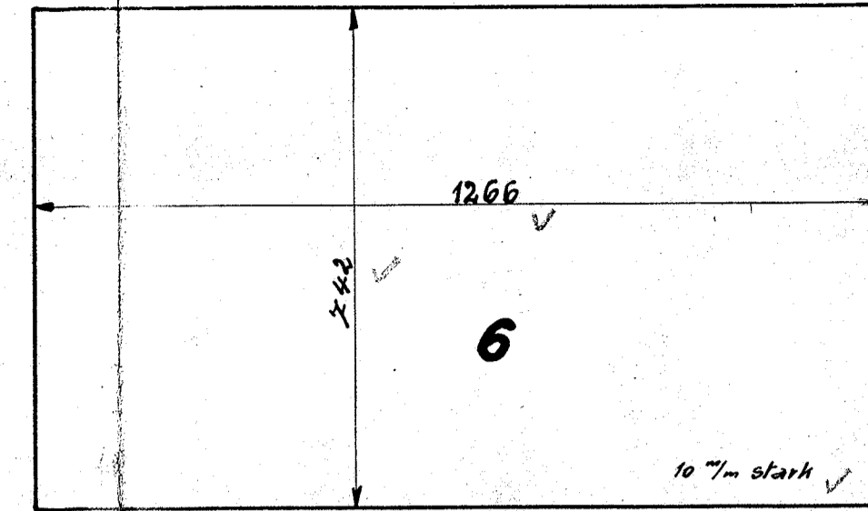
Wasserkasten hinterwand
