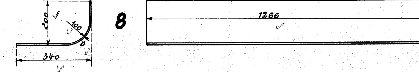
Wasserkastendecke hinten
