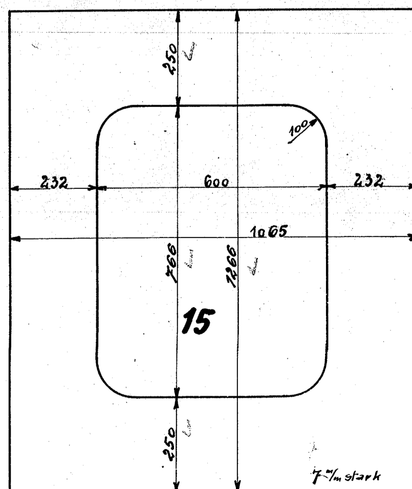
Strebe unter Rauchkammerträger
