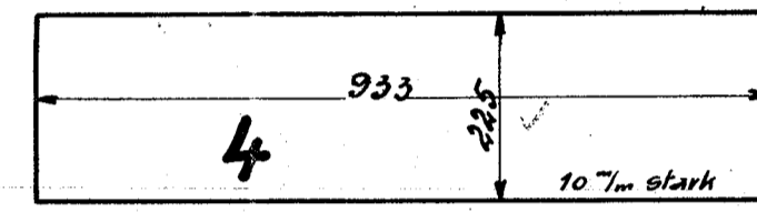
Strebe zw. Laufachse u. Feuerkasten für Bremszylinder
