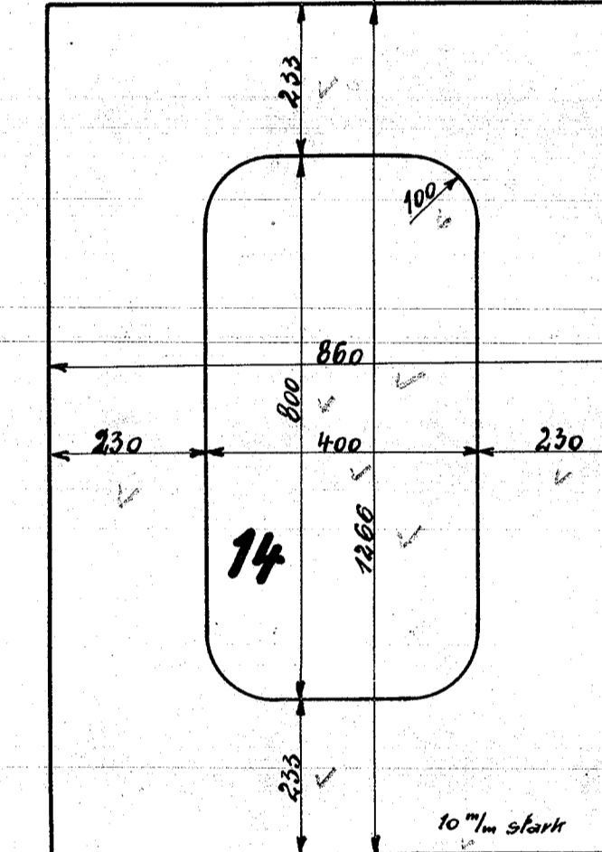
Unt. Cylinderverstrebung
