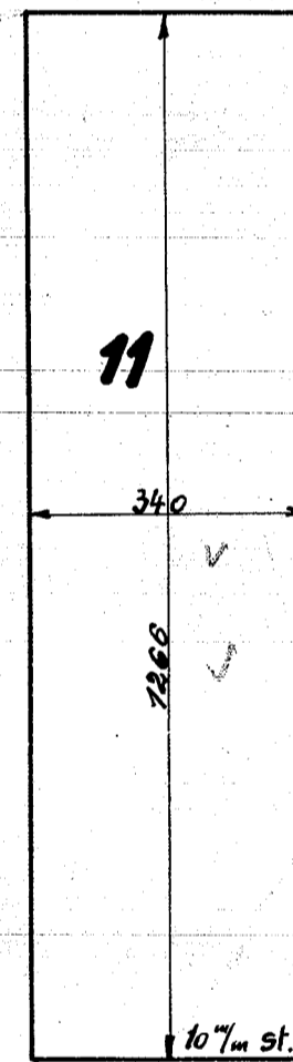
Strebe für vord. Drehgestell
