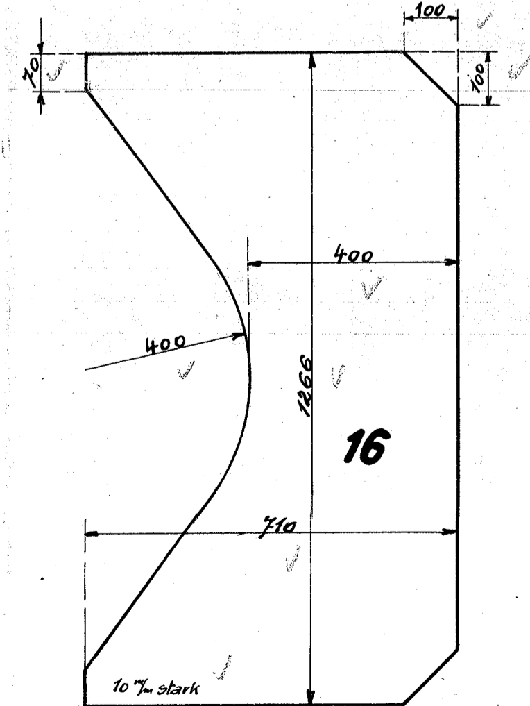
Strebe für vord. Bufferbohle
