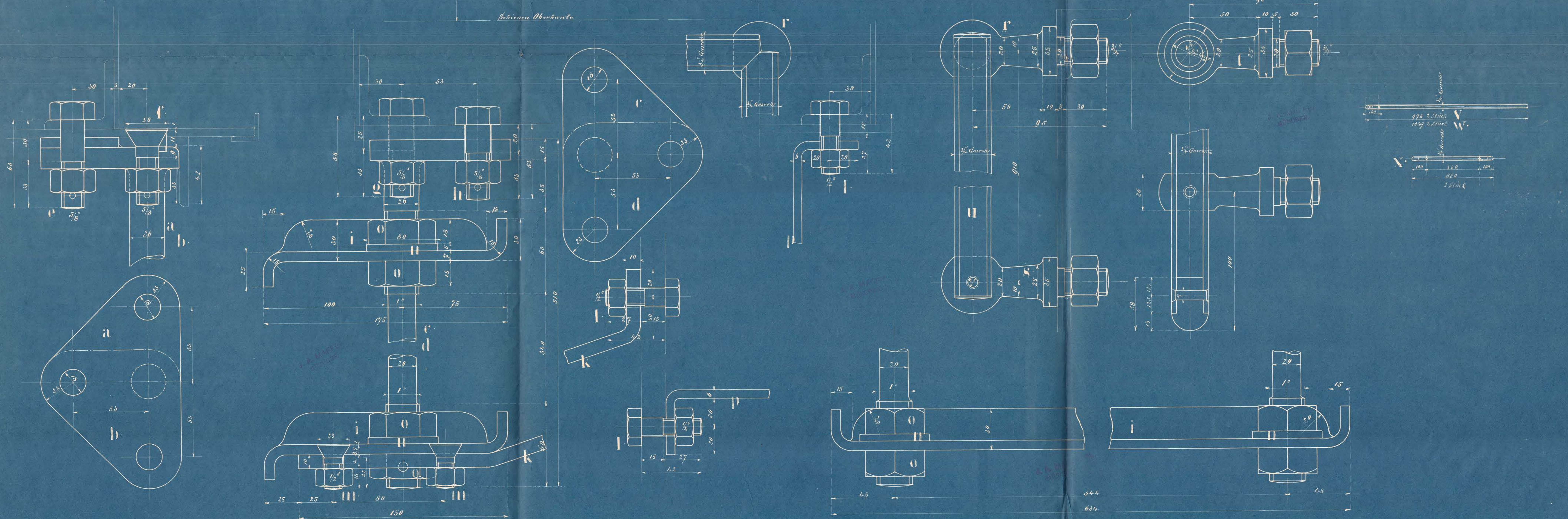
Fußstrille-Luftbehälterbefestigung und Laufstangen.
