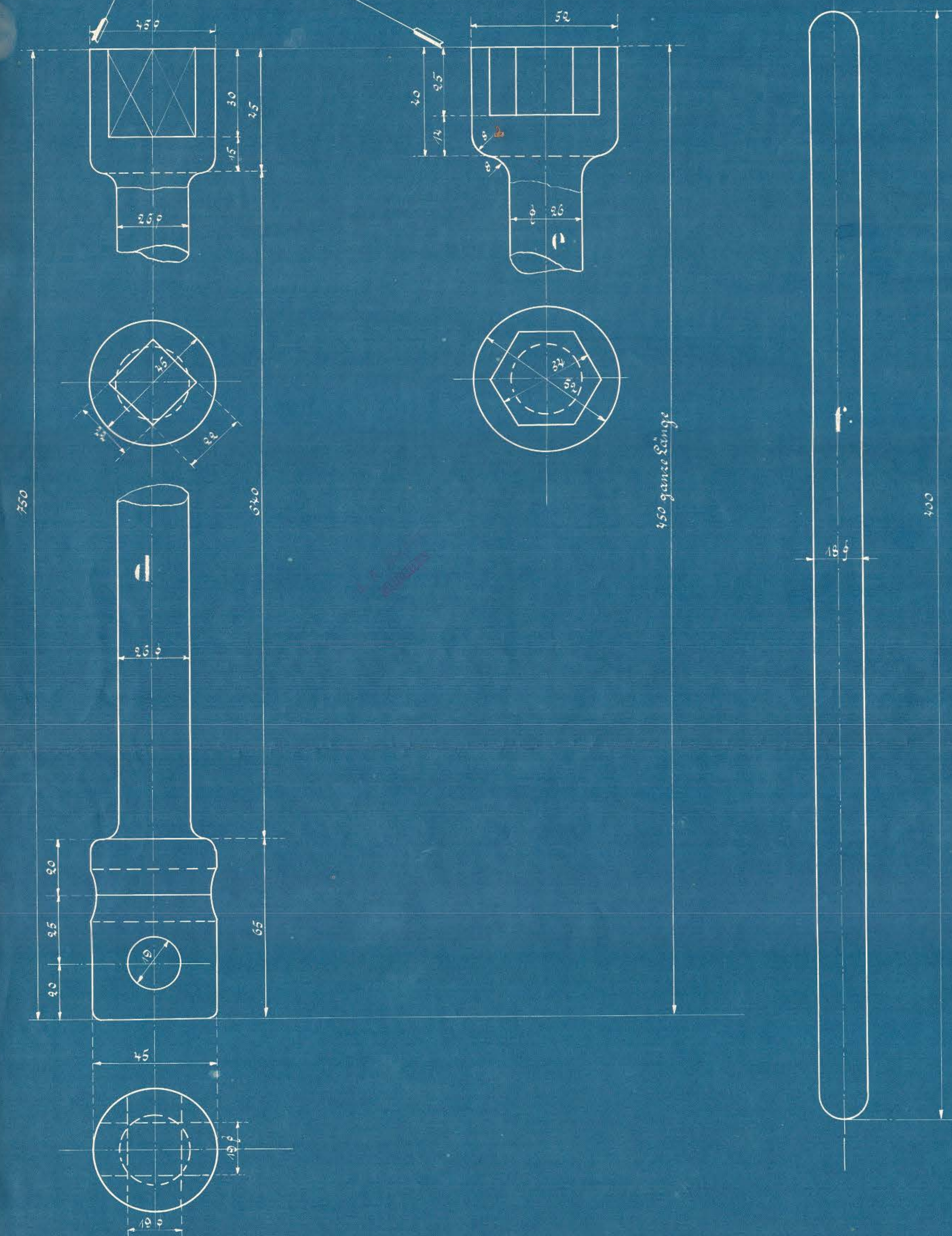
Überhitzer 450lg.
