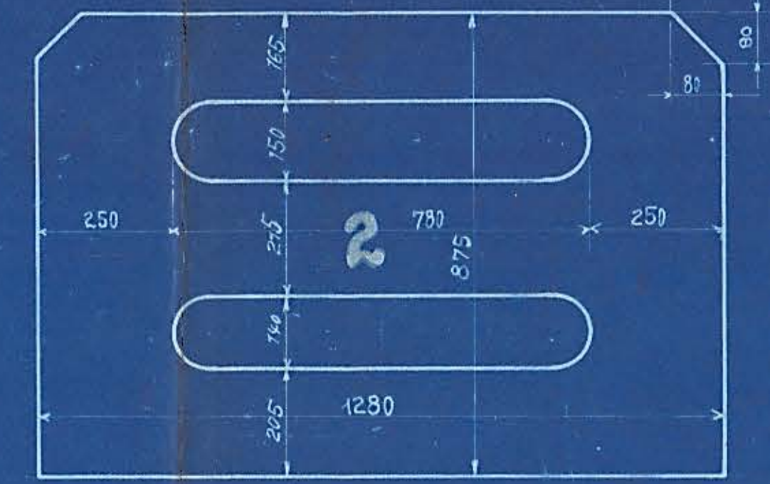
Vertikale Rahmenstrebe hinten, 10 mm stark.
