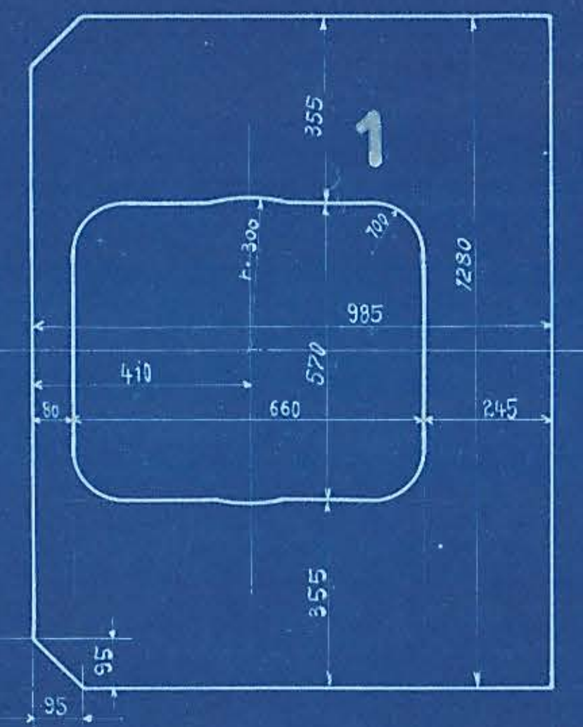
Horizontale Rahmenstrebe hinten, 15 mm stark.
