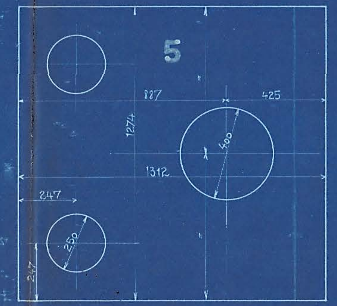
Wasserkastenboden vorn, 6 mm stark.
