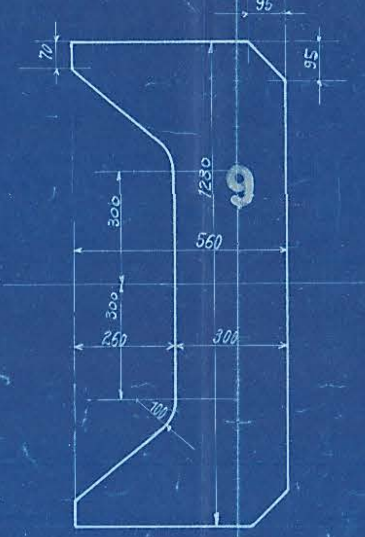
Strebe vorn, 8 mm stark.
