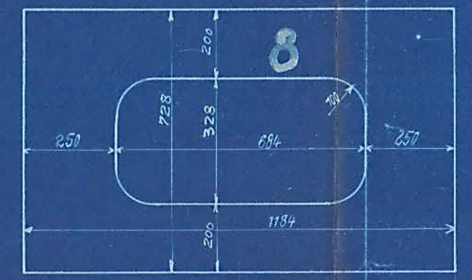
Strebe für Zwischenrahmen 8 mm st.
