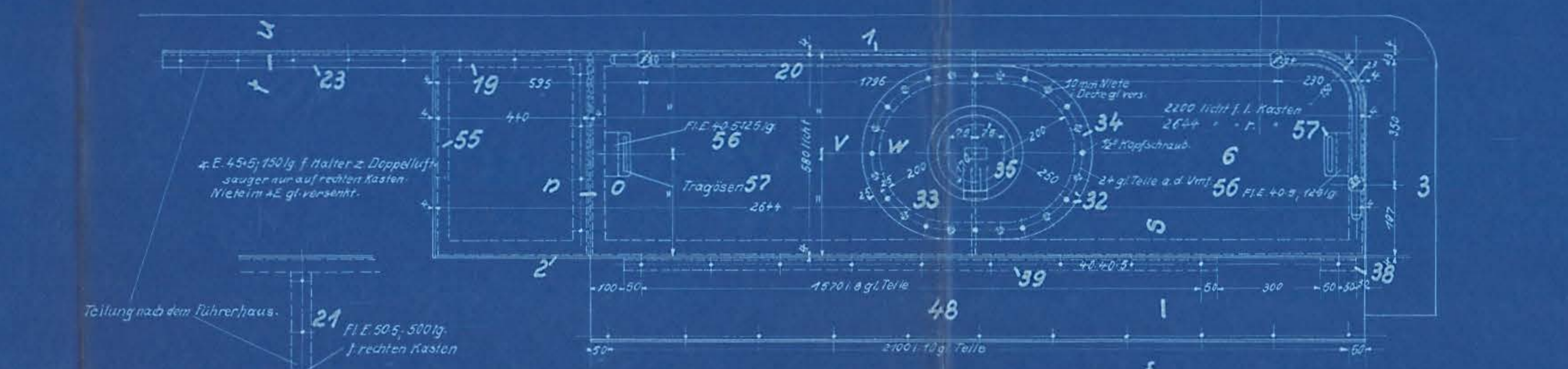
Schnitt c-d
