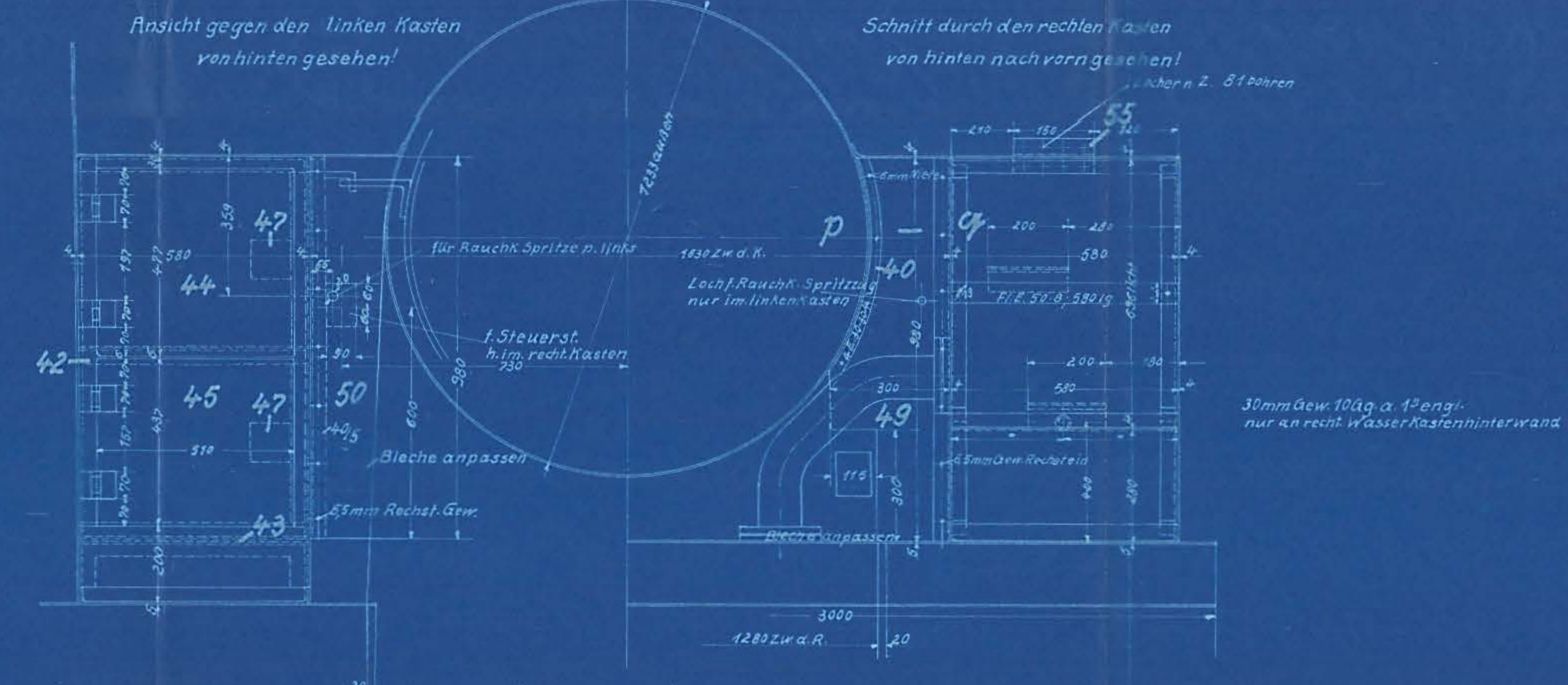
Schnitt a-b
