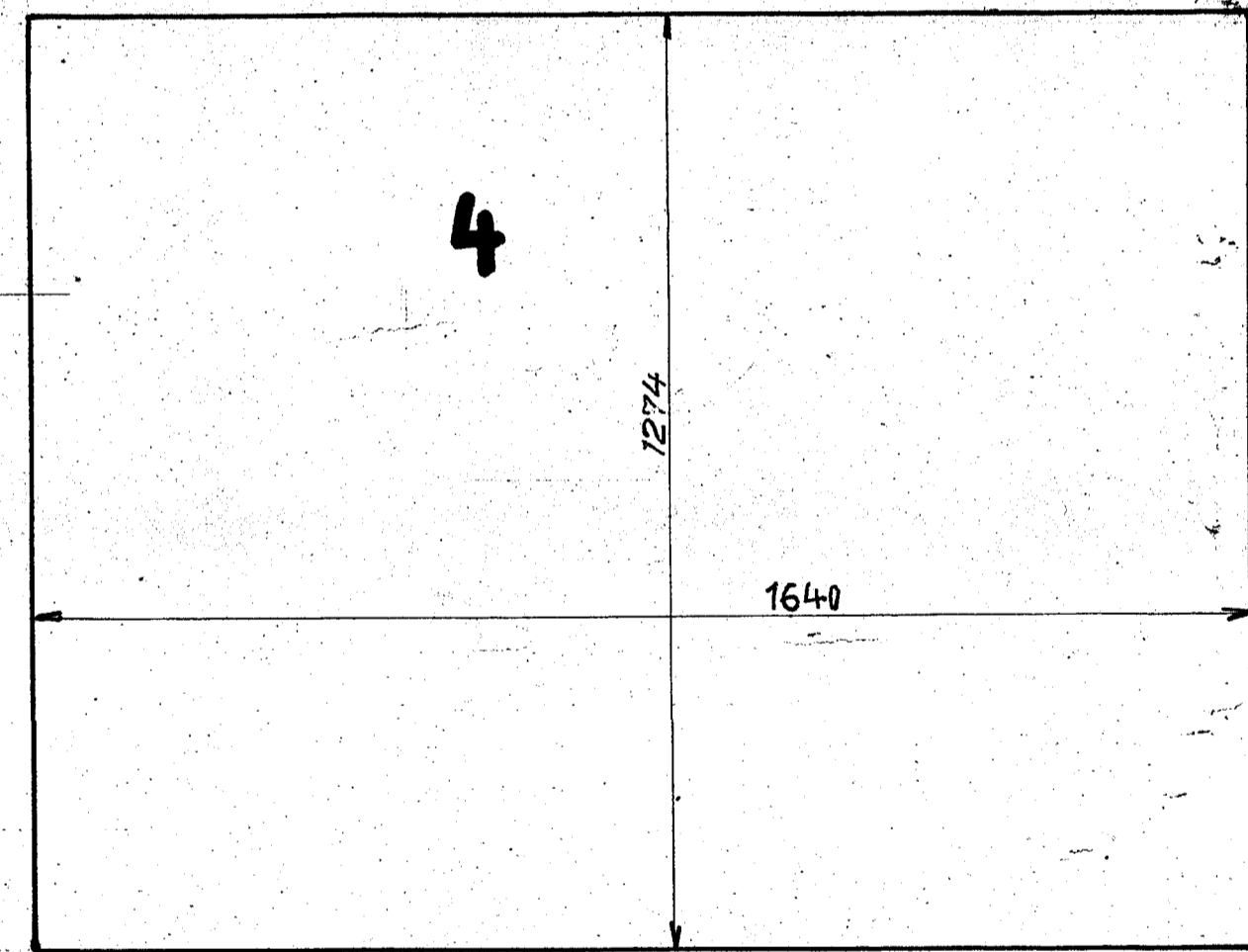
Wasserkastenboden hinten, 6 mm st. gestreckt gezeichnet
