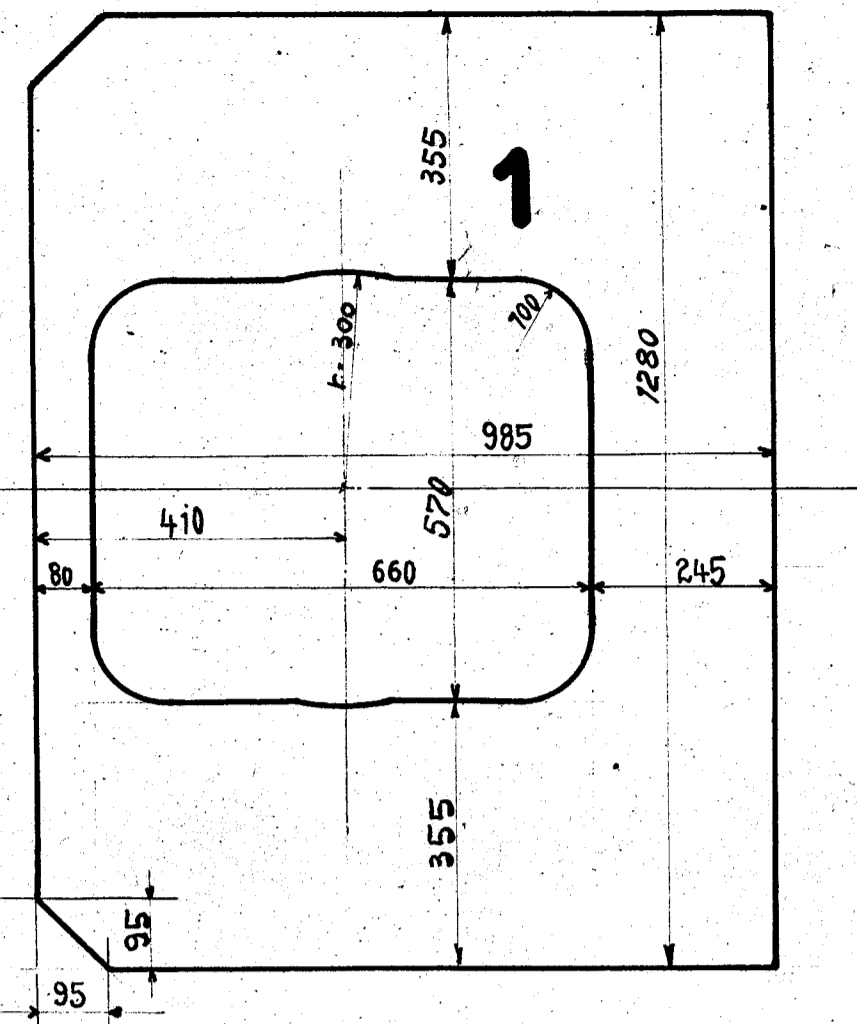
Horizontale Rahmenstrebe hinten, 15 mm stark.
