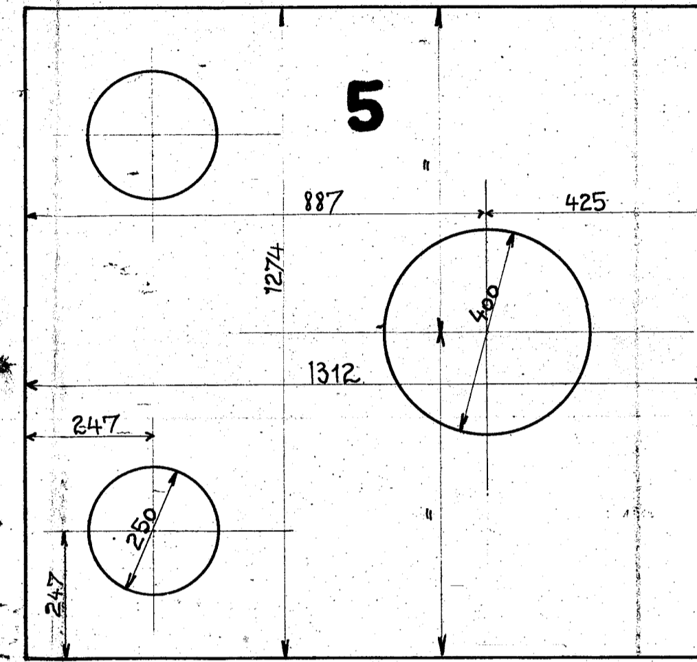
Wasserkastenboden vorn, 6 mm stark
