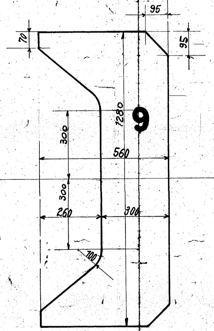
Strebe vorn 8 mm stark.
