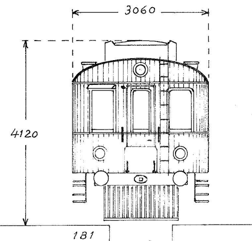
Diesel-hydraulisk „Nakskov-Nydquist/Holeby“, prøve kørt 1927-28 på NPMB uden held, kom ikke i regelmæssig drift. 8 cyl., 215×260 mm, 200 hk, 500 %/m. Tegnet på spinkelt grundlag, eneste foto: DJK 5 s. 17.
