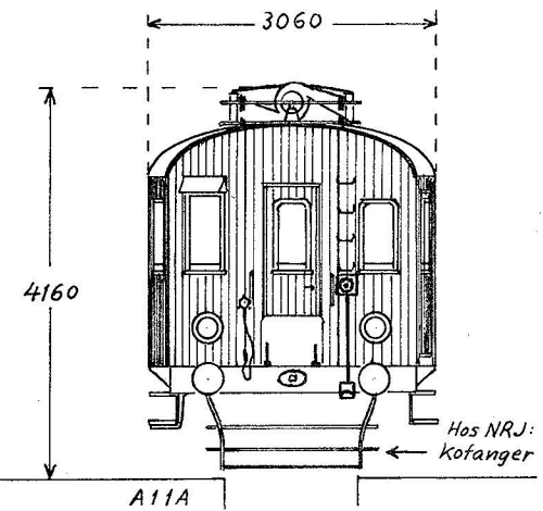
VaGJ M og NRJ M 4 og 5 Diesel-elektrisk post- og rejsegodsvogn. Nakskov/Holeby 1926, 6 cyl. 215×260 mm Effekt 150 hk ved 500 %/m
