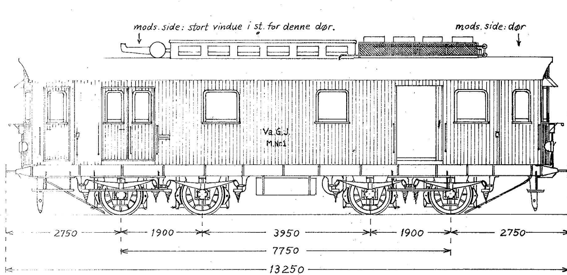
VaGJ M og NRJ M 4 og 5 Diesel-elektrisk post- og rejsegodsvogn. Nakskov/Holeby 1926, 6 cyl. 215×260 mm Effekt 150 hk ved 500 %/m
