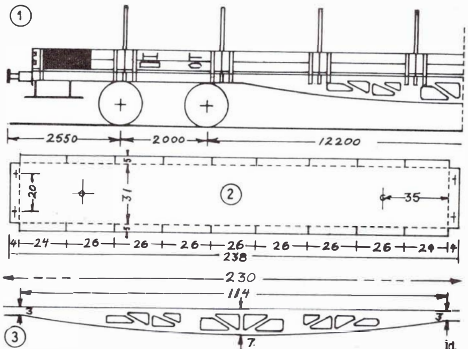
Arbejdstegning 1, 2 og 3 til en T g -vogn
