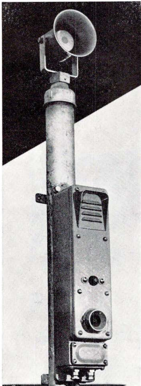
Fig. 5. Højtalon, d.v.s. højtalende telefon. Øverst kaldehøjtaleren; nederst apparatenhed indeholdende forstærkere, mikrofoner, højtalere og kaldeknop.
