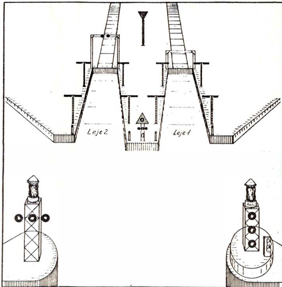
Fig. 14. Besejlings signaler for færgehavn og lejer. Fyrlinien markeres af et for- og et bagfyr med topmærker og røde lanterner. I usigtbart vejr lyder tågesirenen på østre molehoved.
