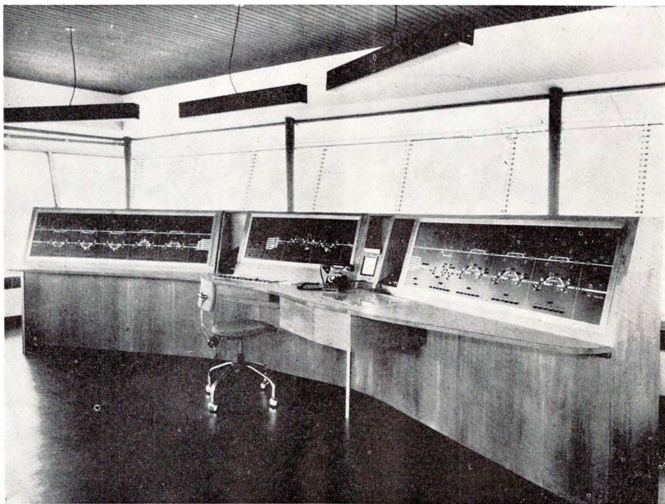
Fig. 12. Centralapparat for fjernstyringsanlæggene Vordingborg-Rodby F og Nykøbing F-Gedser. I bordfladen til venstre for telefonen ses betjeningsapparat for den „automatiske stationsdrift“. Til højre herfor ses togtidsskriveren, der automatisk trykker den grafiske køreplan, der svarer til togenes kørsel.
