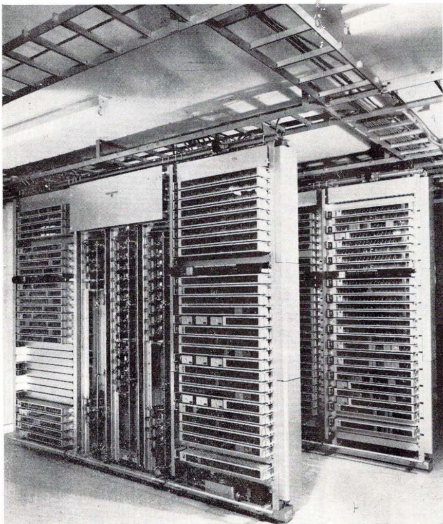
Fig. 4. Knudepunktcentral, Nykøbing F. Venstre stativrække er centralens lokalpart, der formidler telefontrafikken hørende til stationens lokale net samt forbindelsen med det offentlige net. Højre stativrække er fjernparten, der dels forbinder lokalparten med DSB's eget automatiske fjerntelefonnet, dels fungerer som transitcentral i dette net. Tilsvarende knudepunktcentral findes bl. a. på Rødby Færge station, hvor der bl. a. er direkte forbindelse med Brundsbahns central i Puttgården.
