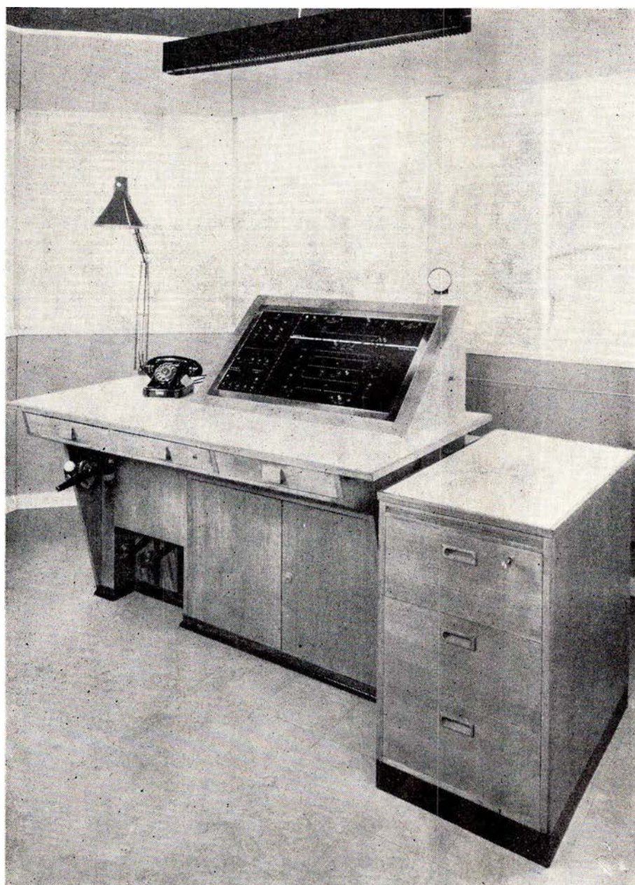
Fig. 13. Centralapparat for Frederik d. 9.'s bro. Fra apparatet manøvreres broklapperne; endvidere sker betjeningen af signaler, bomme m. v. herfra. Nederst til venstre ses betjeningshåndtag for broklappernes nødmanøvrering ved hjælp af en dieselmotor.
