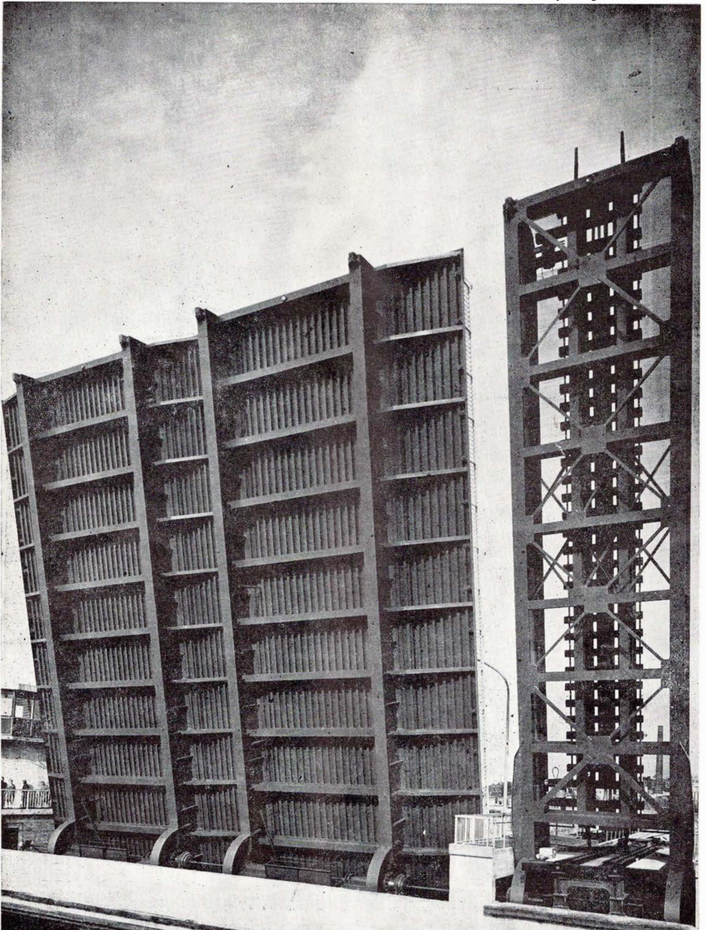
DOBB. KLAPBRO OVER GULDBORGSUND Frederik d. IX Bro, leveret til De Danske Statsbaner
