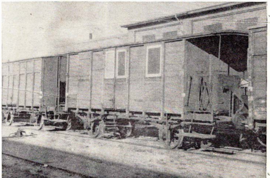
En af de veltjente bænkevogne G 75
