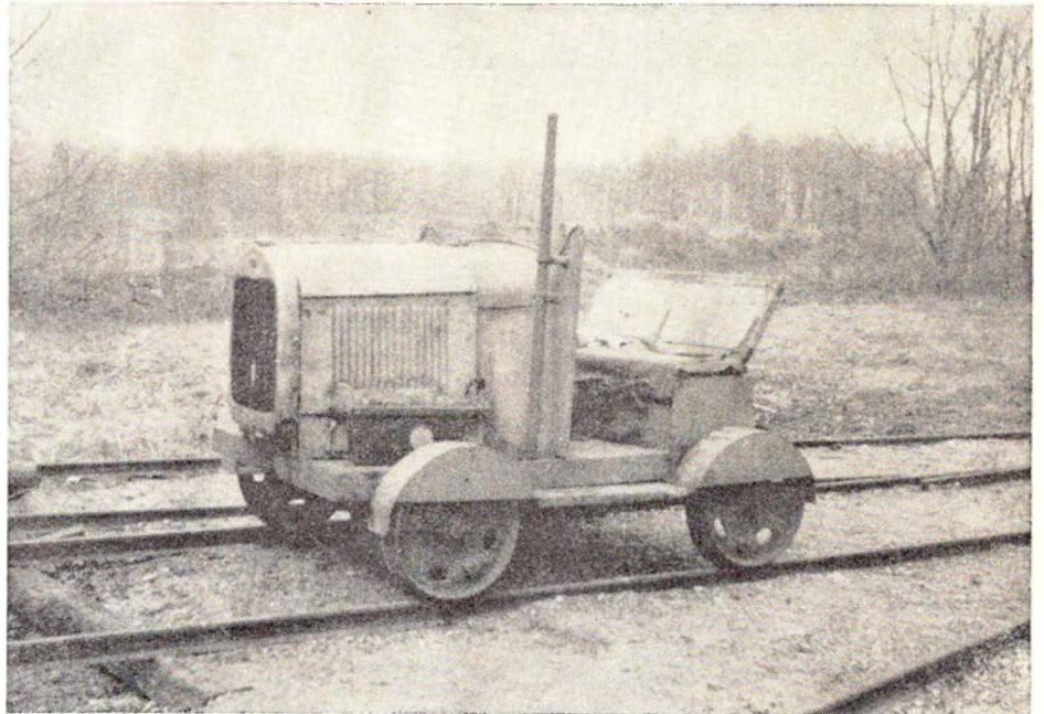
Banemester Mikkelsens motortrolje, ETJ, Skærsø
