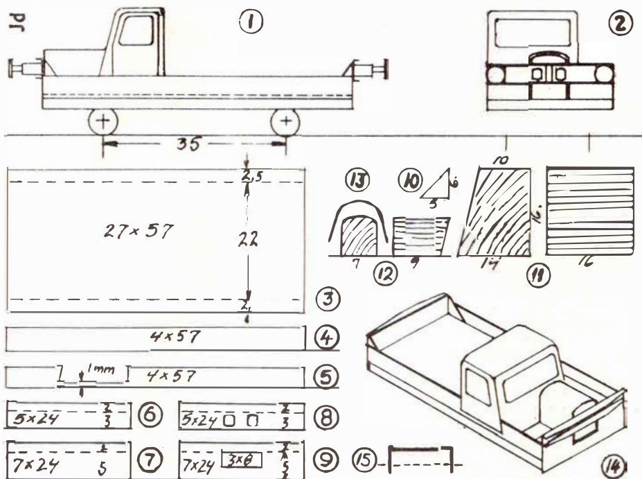
Arbejdstegning til en motertrolje
