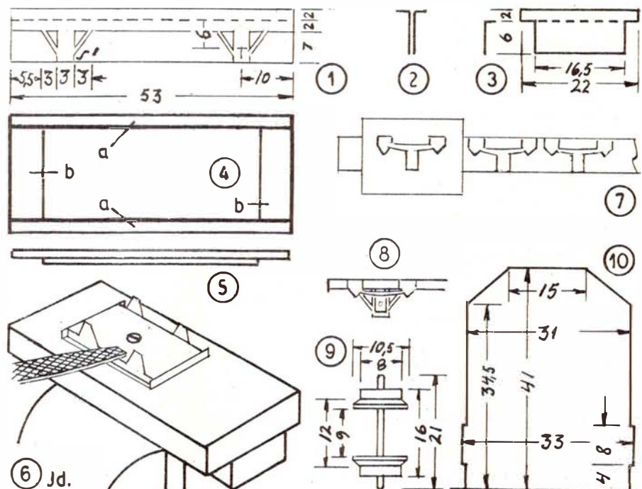
Arbejdstegning til smalsporvogne
