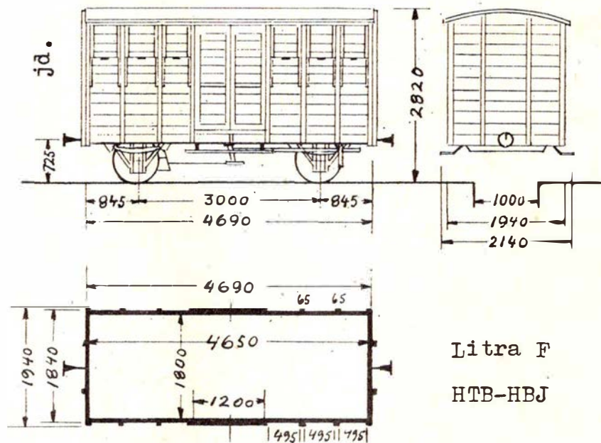
Arbejdstegning til smalspor godsvogn
