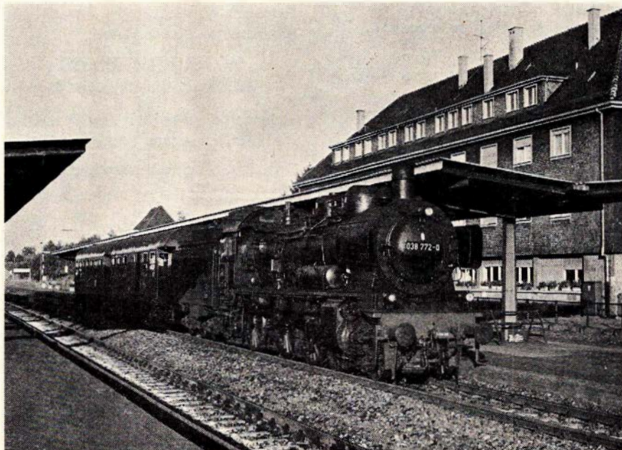
Deutsche Bundesbahn's sidste P8'er med persontog i Eutingen. Foto: -tl-.
