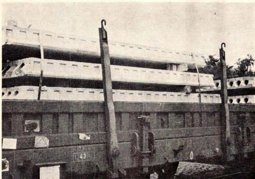
Dækelementer i lavsidet åben godsvogn.
