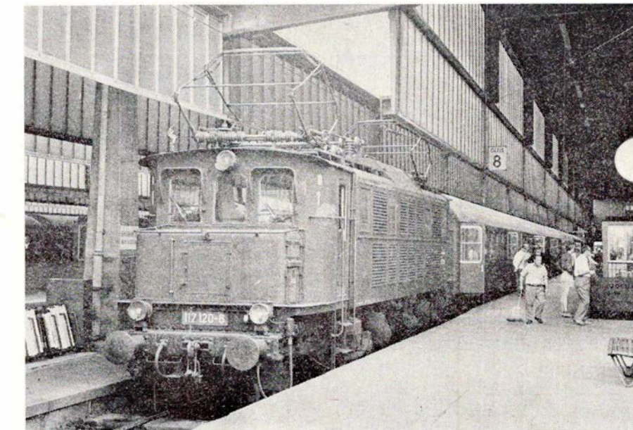
DB 117.120-6 på hovedbanegården i Stuttgart i 1969. Det er bygget i 1929 af Siemens og AEG.
