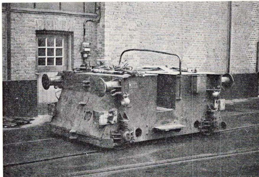
Akkumulatorlokomotiv hos A/S Frichs, Århus.
