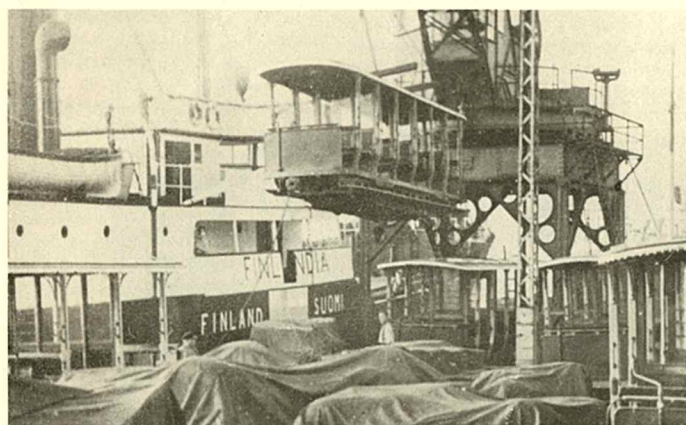
Fig. nr. 6. Åbne bivogne bliver lastet til »Helsingfors Spårvägar«.
