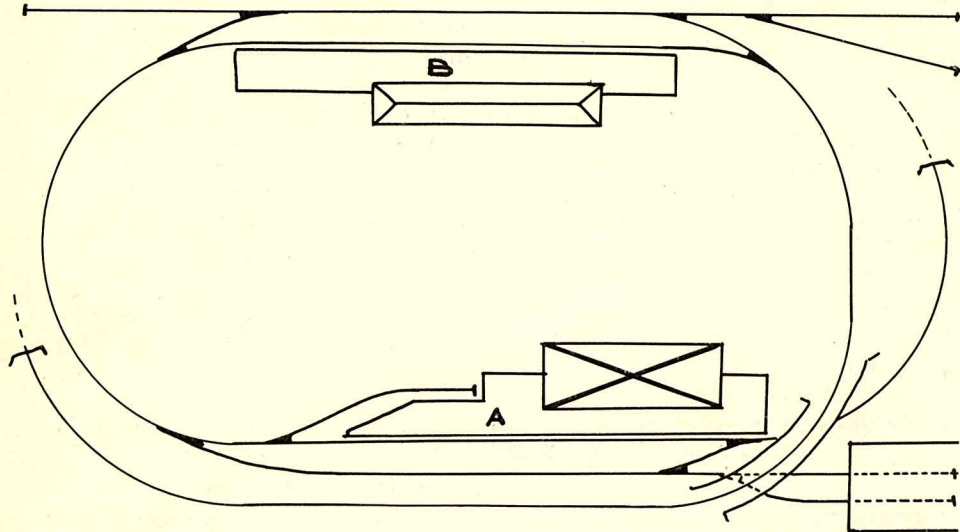
Plan 3: viser et såkaldt 8-tal. Vi har valgt at »lægge det sammen«, således at den ene cirkel går under station A i en tunnel. Herved har man opnået en lang bane på et forholdsvis lille område. Banen måler i HO (1:87) 1,10x2,00 m.
