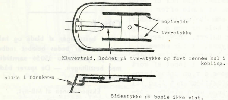
Fig. 3. (Koblingens anbringelse)
