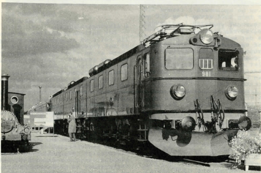
Øverst: Det nye rød-hvid-blå stribede T-43 dieselloko, der leveres i et antal af 50 stk. til afløsning af damplokomotiverne på ikke elektrificerede strækninger. Nederst: 3-leddet malmtogslokomotiv litra DM 3, længde 32,25 m, effekt 9 000 HK.
